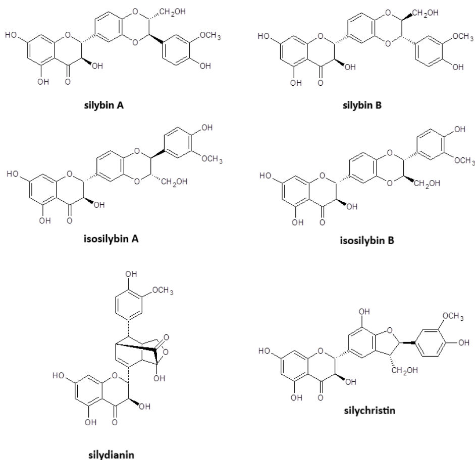
Obr. 5 Strukturní vzorce jednotlivých složek silymarinu (silybin A a B, isosilybin A a B, silydianin, silychristin) (upraveno podle Kumar et al. , 2011).
