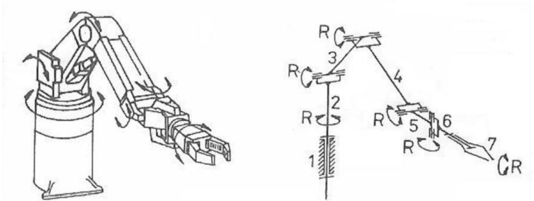
Obr. 36) Schéma robotu [27]
