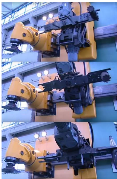
Obr. 35) Vyklopení manipulátoru [24]
