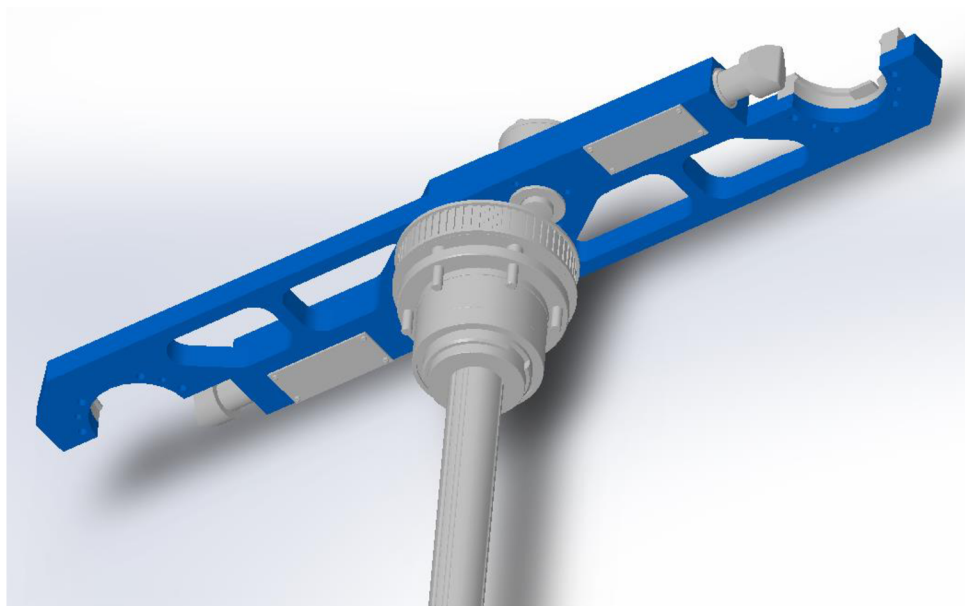
Obr. 18) Odlehčené tělo ramene
