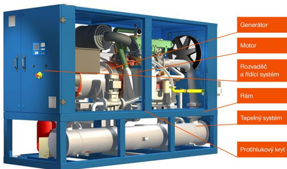
obr. 6: Kogenerační jednotka [27]
