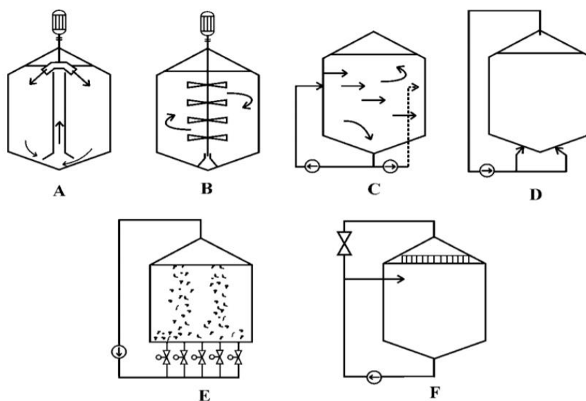
obr. 3: Základní typy míchadel [23]
