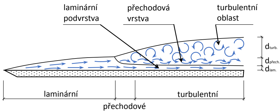
Obr. 2 - Mezní vrstva
