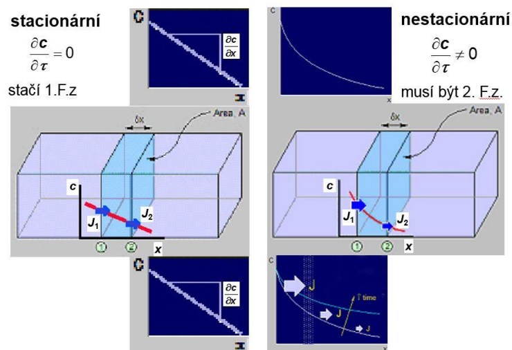
Obr. 8 - Difuze stacionární, nestacionární 9
