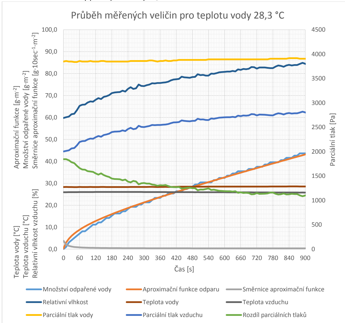
Graf 17 - Měřené veličiny pro teplotu vody 28,3 °C
