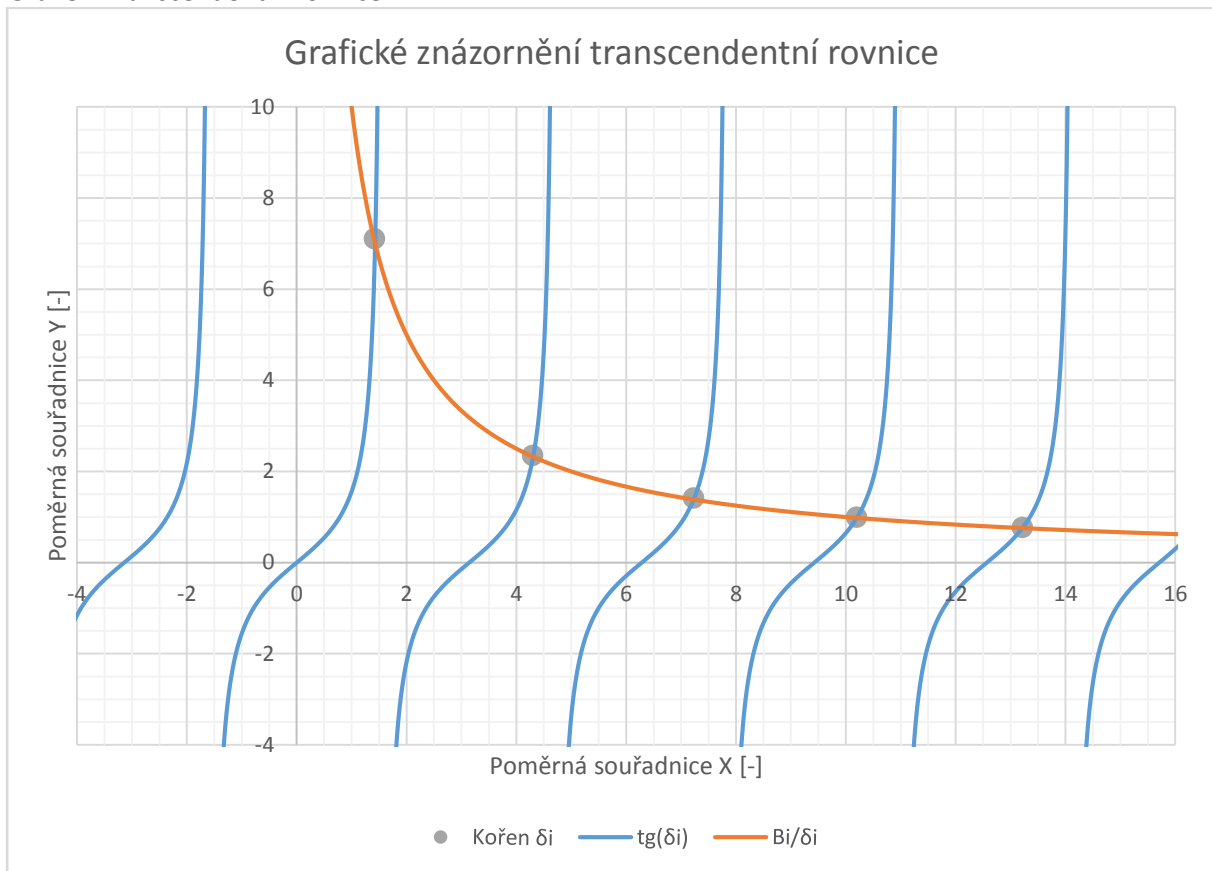
Graf 3 - Transcendentní rovnice
