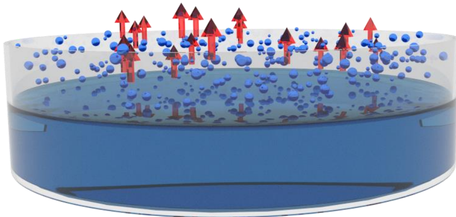
Obr. 10 - Odpar z vodní hladiny
