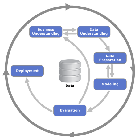
Obrázek 2.2: Model CRISP-DM [8]
