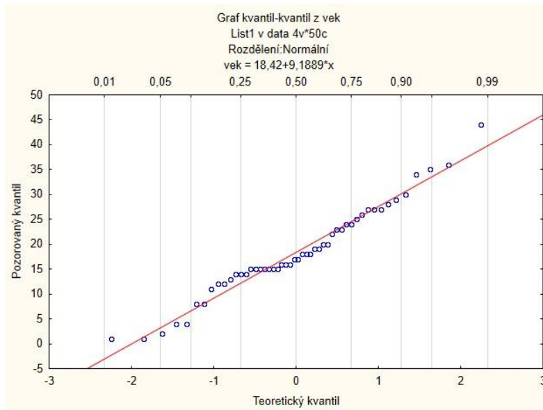
Obrázek 7 Q-Q graf 1
