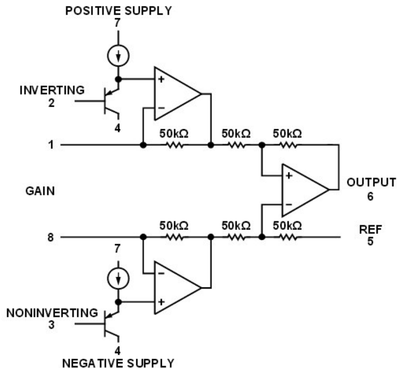
Obr. 2.5: Zjednodušené vnitřní zapojení přístrojového operačního zesilovače AD623 (převzato z [4]).
