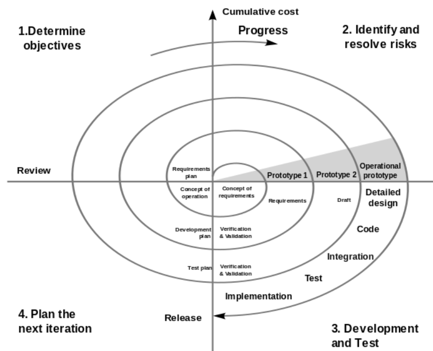
Obrázek 3 - Spirálový model
