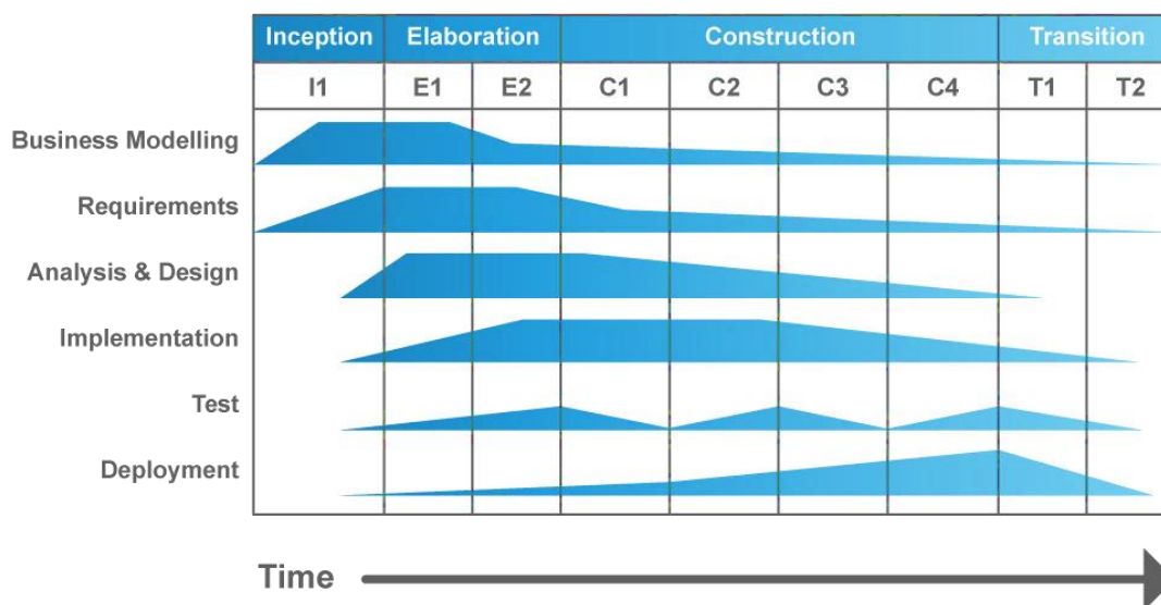
Obrázek 4 - RUP
