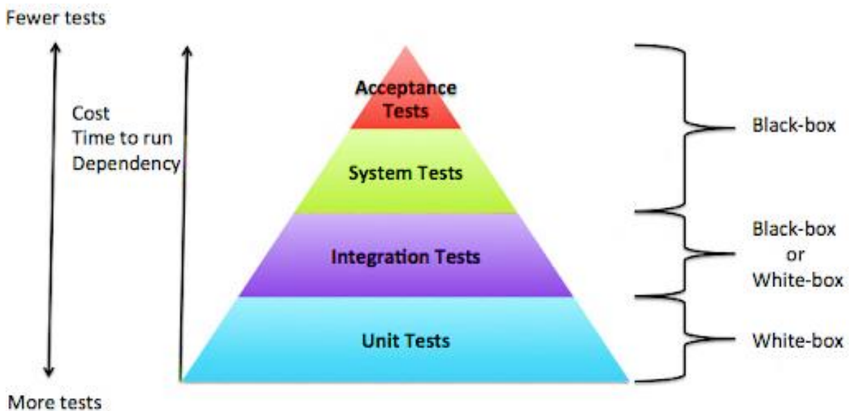
Obrázek 7- Testovací fáze
