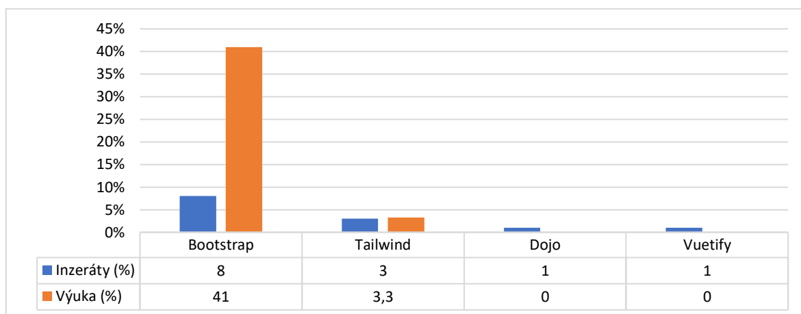
Obrázek 61: Porovnání CSS frameworků
