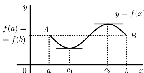
(a) Rolleova věta
