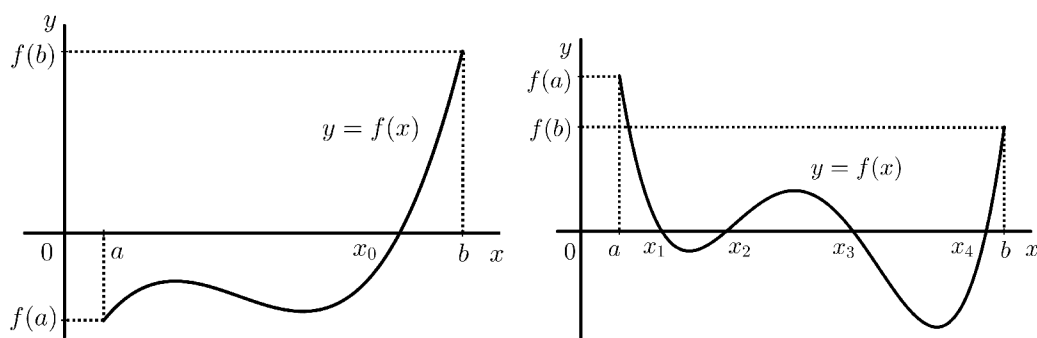
Obrázek 2.4: Bolzanova věta.
