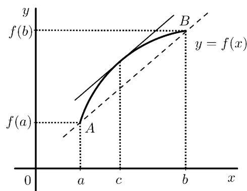
(b) Lagrangeova věta
