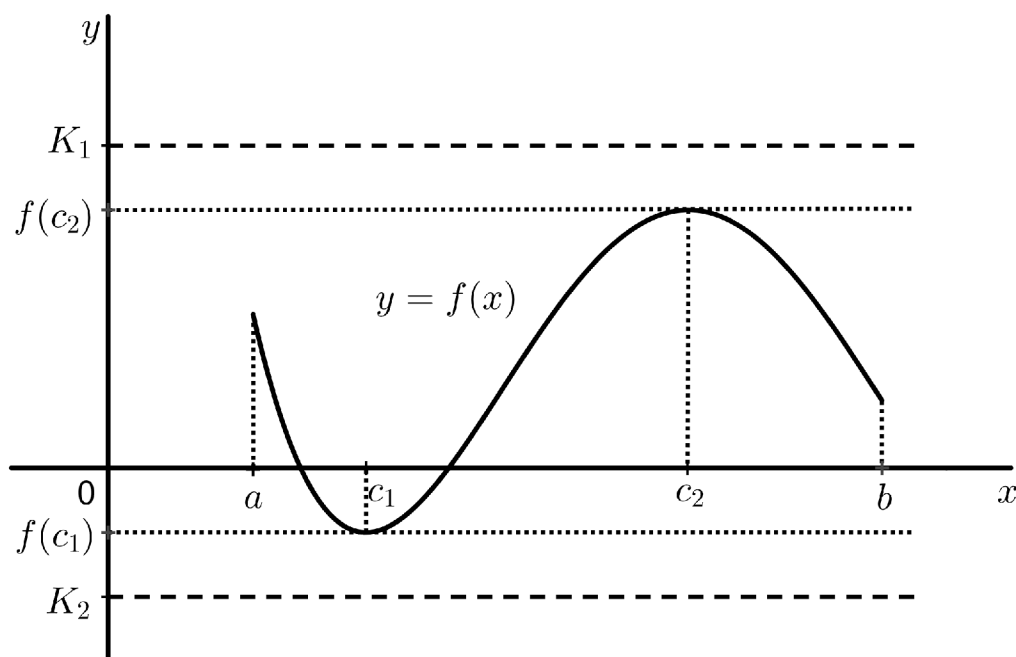
Obrázek 2.3: Weierstrassova věta
