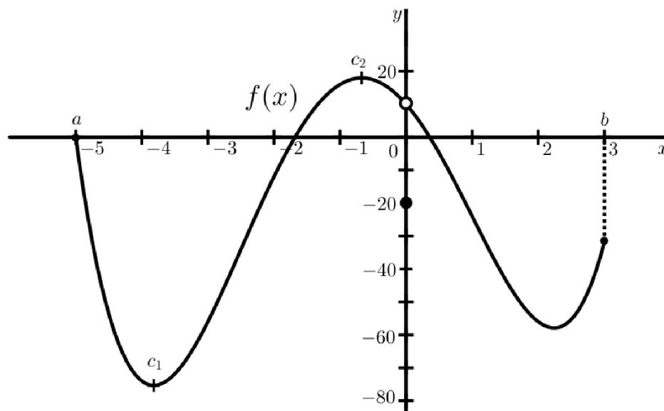
Obrázek 2.5: Funkce f(x) = \begin{cases} x^4 + 3x^3 - 15x^2 - 23x + 10, & \text{pro } x \in \langle -5, 0 \rangle \cup (0, 3 \rangle \\ -20, & \text{pro } x = 0. \end{cases}
