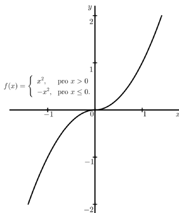
Obrázek 3.11: Funkce f(x) = \begin{cases} x^2, & \text{pro } x > 0 \\ -x^2, & \text{pro } x \leq 0. \end{cases}
