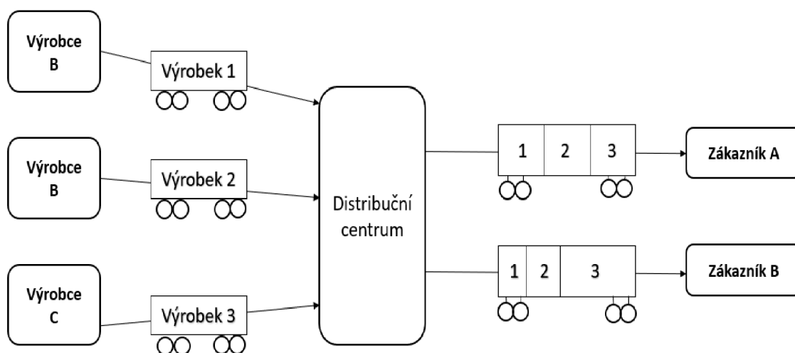
Obr. 1.9 Princip kompletace
