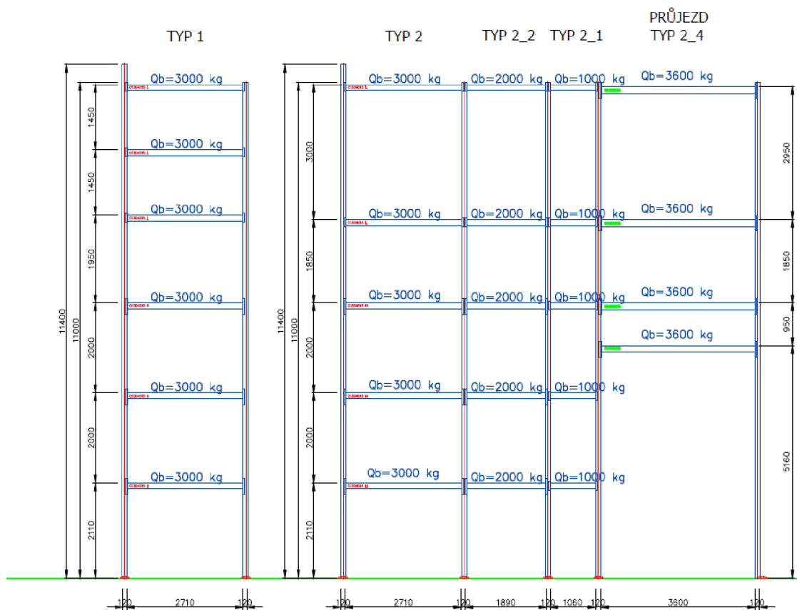
Obr. 2.15 Regálový systém suchého skladu FOOD
