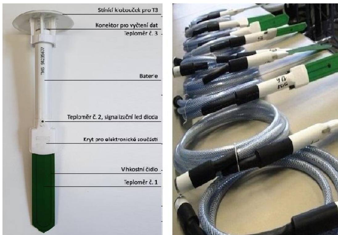
Obrázek 11: Sonda TOMST TMS-4 s popisem a Obrázek 12: Vlhkostní sonda TOMST TMS-4 osazená kabelem pro zakopávání (zdroj: Tomst s.r.o., upravil autor 2022).
