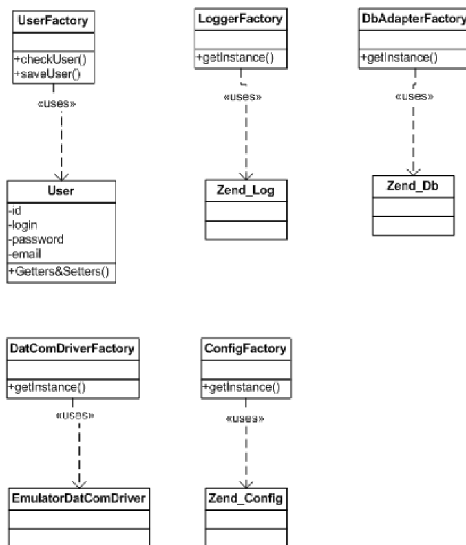
Obrázek A.1: Diagram návrhových tříd zobrazovacího systému.
