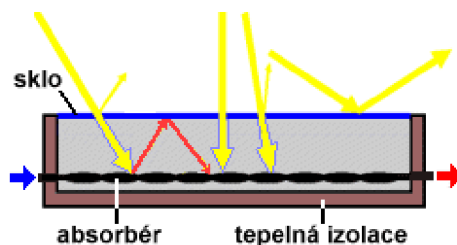
Obrázek 2.2: Schéma konstrukce běžného kolektoru (převzato z [4]).
