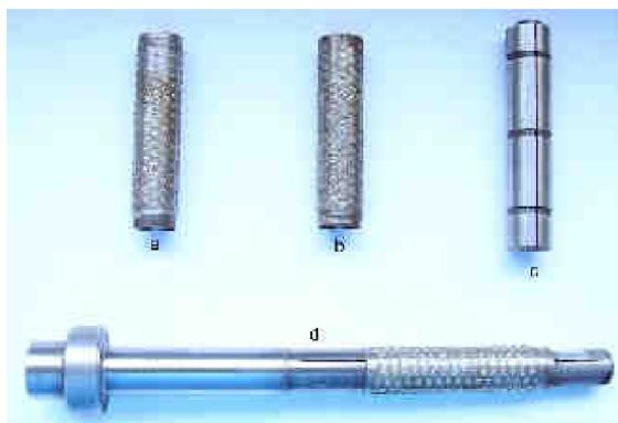
Obr. 2.3 Pouzdra pro obrábění hlavního otvoru průměr 12 mm: a) střední, b) jemné, c) lapovací pouzdro d) nosič s hrubým pouzdrém
