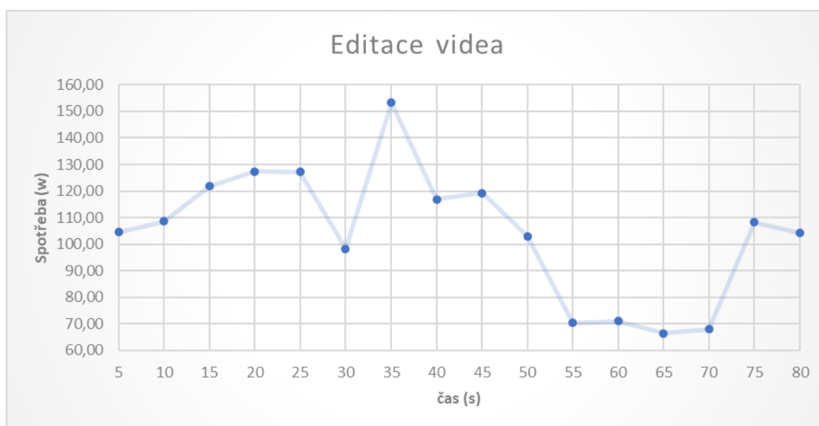
Obrázek 12: graf zobrazující průběh spotřeby při editaci videa u PC č.2
