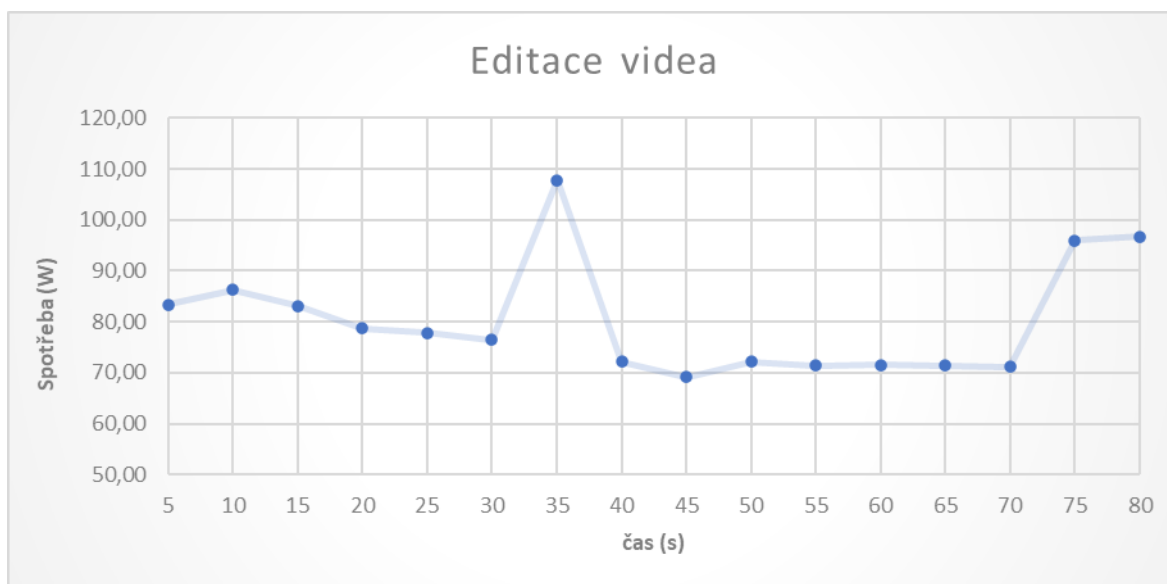
Obrázek 16: graf zobrazující průběh spotřeby u editace videa u PC č.3 Zdroj: [vlastní tvorba]
