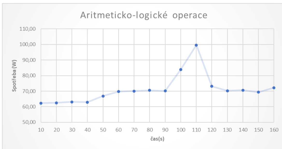
Obrázek 7: graf zobrazující průběh spotřeby při aritmeticko-logických operacích u PC č.1 Zdroj: [vlastní tvorba]
