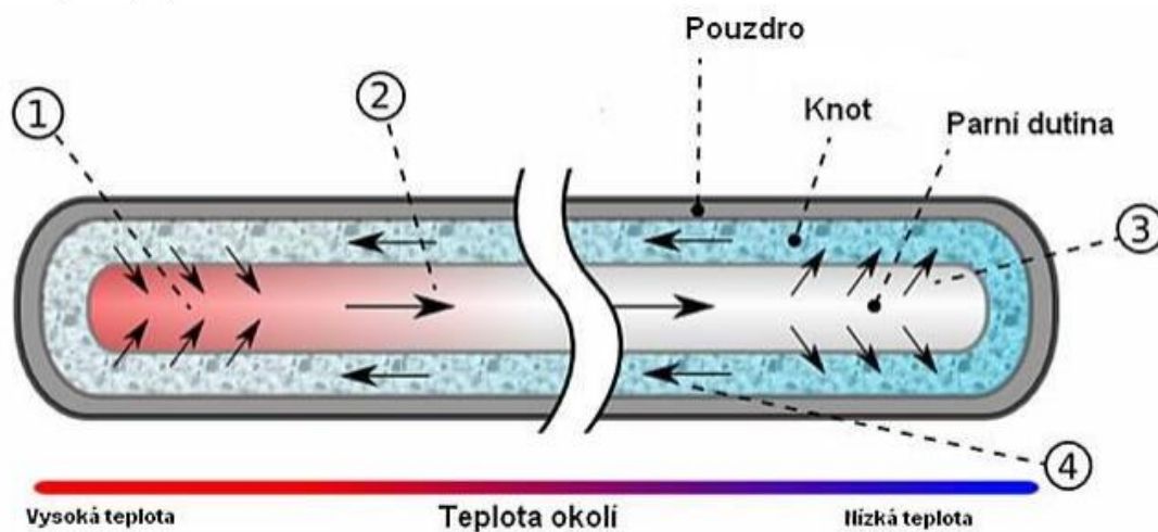
Obrázek 2: Schéma heatpipe
