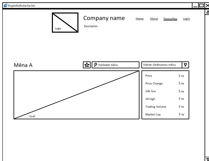
Obrázek 5: Návrh uživatelského rozhraní
