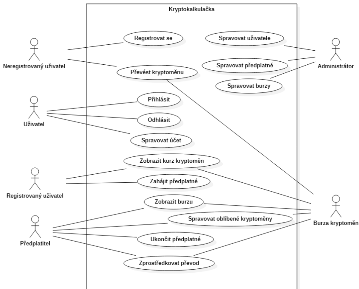
Obrázek 25: Diagram případů užití - kryptokalkulačka.
