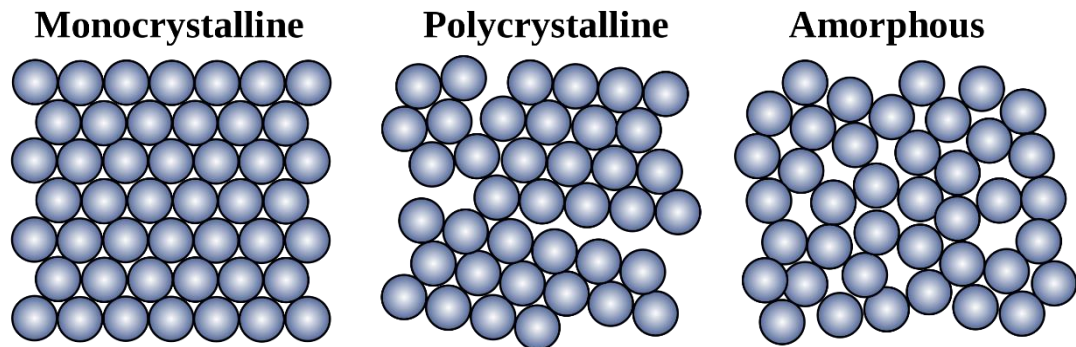
Obr.13 Schéma alotropických forem křemíku: monokrystalický křemík, polykrystalický křemík a amorfní křemík [6]
