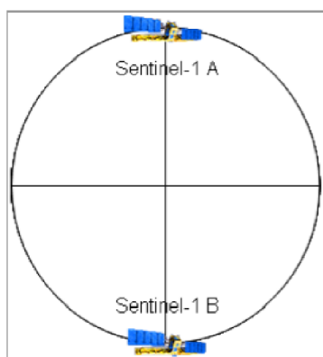
Obrázek 9 Konstelace družice Sentinel 1A a 1B (23)
