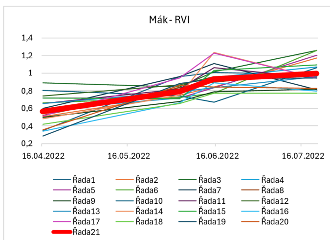
Obrázek 29 Hodnoty RVI pro porost máku v čase, Řada 1 až 20 – hodnoty indexu v jednotlivých bodech v rámci pozemku, Řada 21 – průběh střední hodnoty indexu v rámci pozemku
