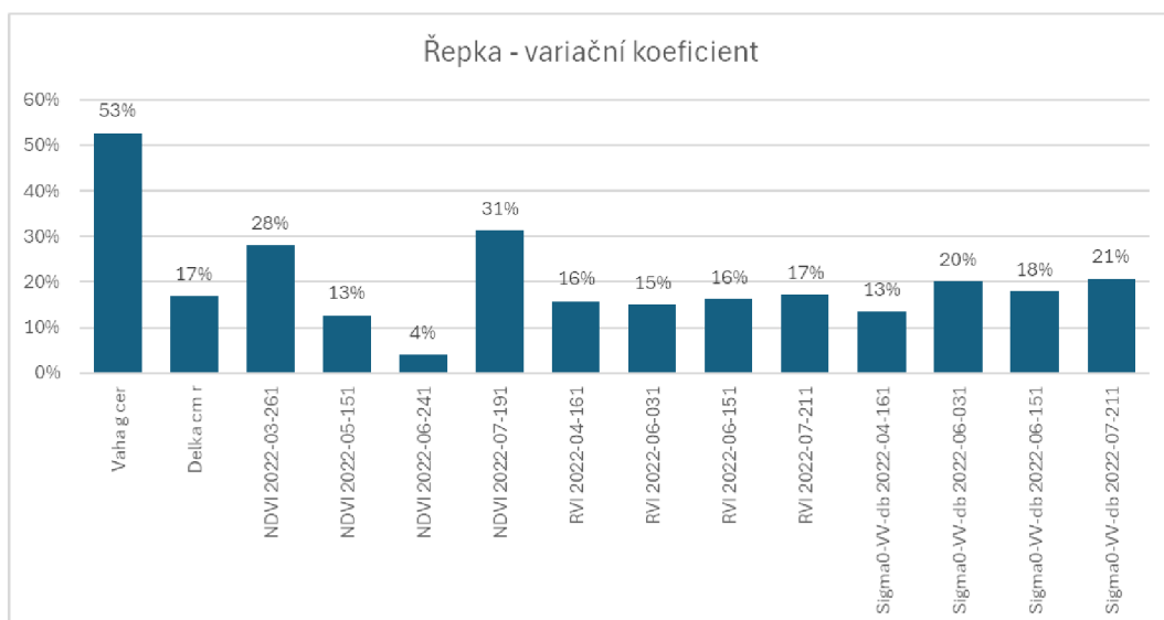
Obrázek 36 Hodnoty variačního koeficientu pro data použitá pro analýzu porostu řepky
