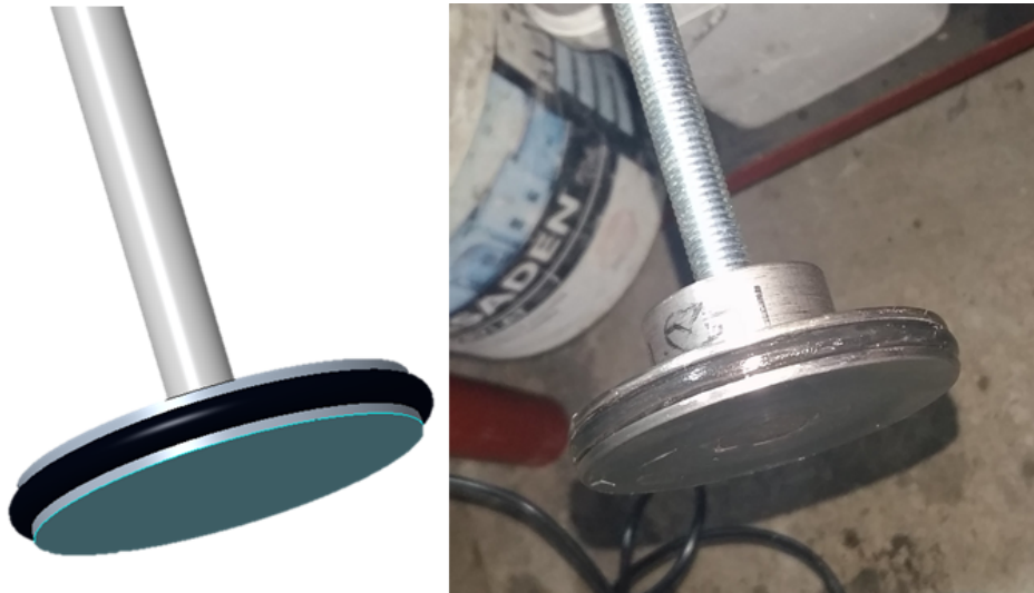
Obr. 17: Model piestika a vyrobený piestik
