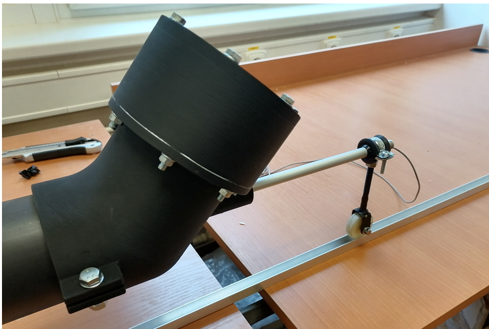
Obr. 18: Mikrofónna sonda
