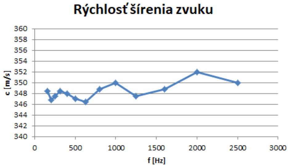
Obr. 28: Rýchlosť šírenia zvuku v impedančnej trubici
