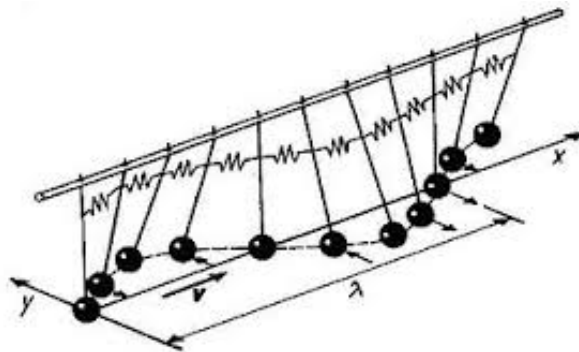
Obr. 1: Priečne vlnenie (prevzaté z [19])
