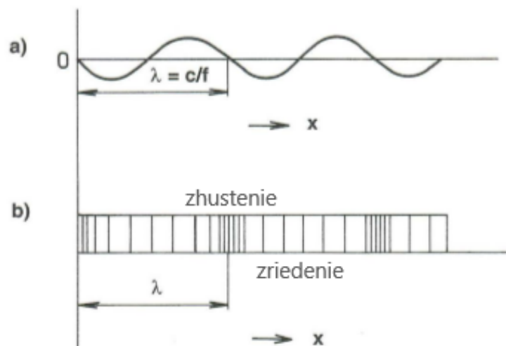
Obr. 6: Zmena hustoty častíc (prekresené z [25])
