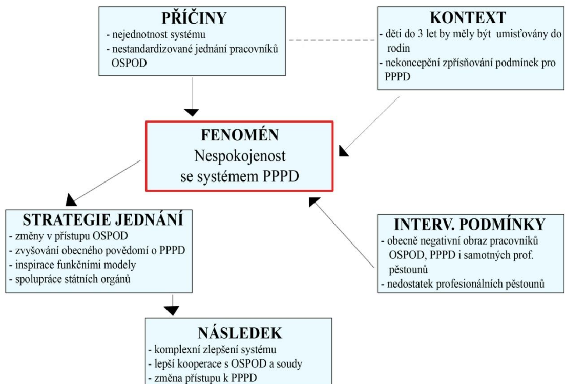
Obrázek 2: Paradigmatický model
