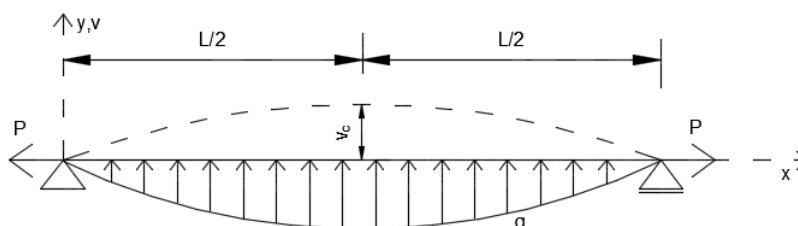
Obrázek 2.1: Prostý nosník
