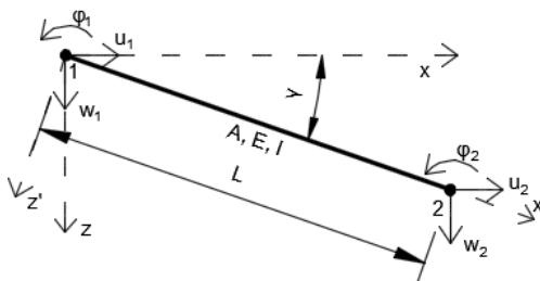
Obrázek 3.1: Oboustranně monoliticky připojený prut
