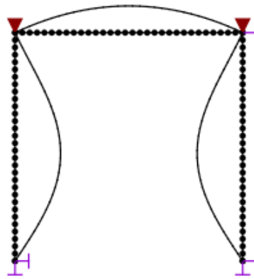
Obrázek 4.27: 90 prvků - P_{cr} = 1083.13107kN
