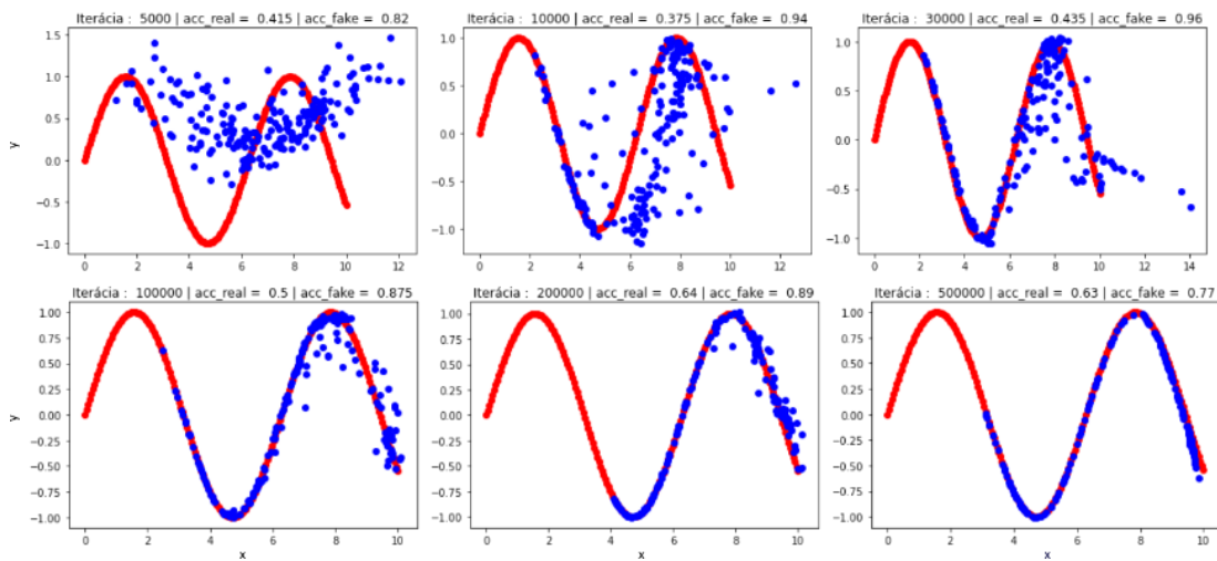
Obr. 5.5: Zobrazenie postupného učenia GAN pre generovanie funkcie sínus s nemennou amplitúdou. Vidíme, že s narastajúcim počtom iterácií sa GAN učí generovať (modré body) podobné vzorky ako reálne dáta (červené body). V názve grafu vidíme v akej iterácii sa GAN aktuálne nachádza a s akou pravdepodobnosťou si diskriminátor myslí, že sa jedná o reálnu (acc_real) a falošnú (acc_fake) vzorku.
