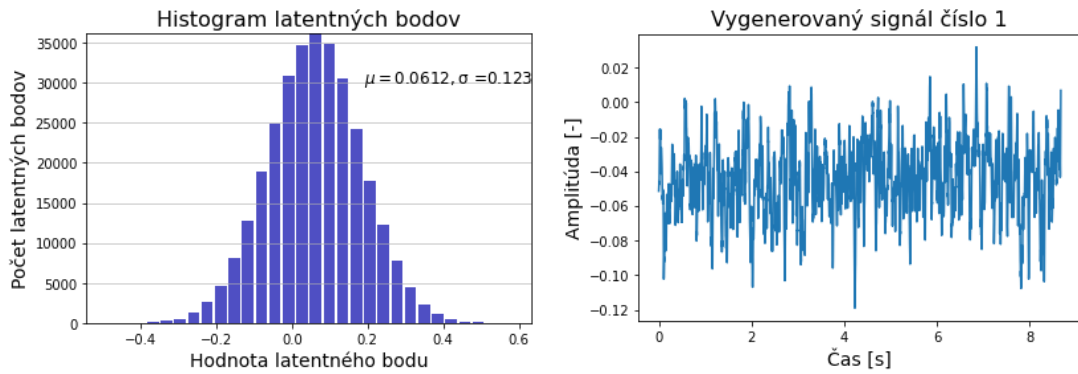
Obr. 4.17: Ukážka generovania signálu z latentných bodov
