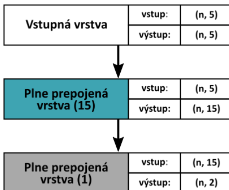
Obr. 4.4: Implementácia (hore) architektúry (dole) generátoru pre generovanie mocninatej funkcie x^2 . V pravej časti každého z troch blokov, ktoré znázorňujú jednotlivé vrstvy generátoru, je uvedený rozmer vstupných aj výstupných dát. Počet neurónov vrstvy je uvedený v zátvorke za jej názvom.
