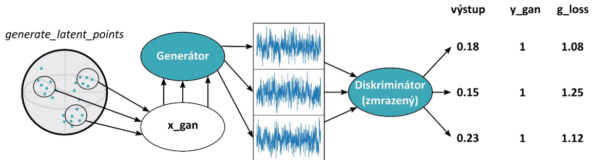
Obr. 4.21: Spôsob tréningovania generátoru na EKG signáloch. Všetky použité obrázky EKG signálov, sú z databázy signálov poskytnutých vedúcim tejto práce.
