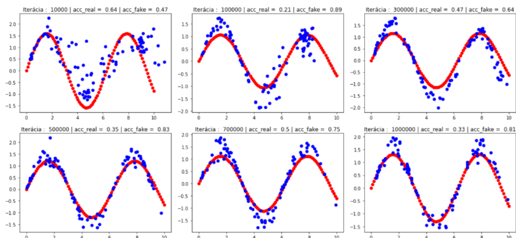
Obr. 5.9: Zobrazenie postupného učenia GAN pre generovanie funkcie sínus s premenlivou amplitúdou. Vidíme, že s narastajúcim počtom iterácií sa GAN učí generovať (modré body) podobné vzorky ako reálne dáta (červené body). V názve grafu vidíme v akej iterácii sa GAN aktuálne nachádza a s akou pravdepodobnosťou si diskriminátor myslí, že sa jedná o reálnu (acc_real) a falošnú (acc_fake) vzorku.
