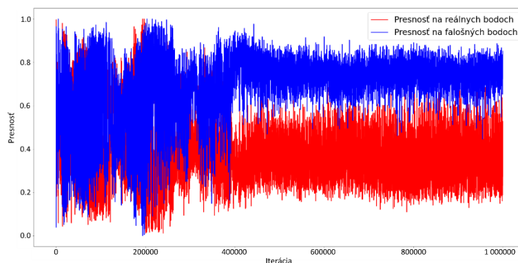
Obr. 5.12: Vývoj presností diskriminátora na reálnych a falošných dátach počas tréningu modelu GAN pre generovanie funkcie sínus premenlivou amplitúdou. Pre lepšiu názornosť je zobrazená len každá 100-tá hodnota presnosti.
