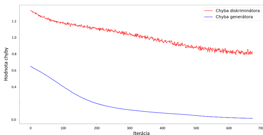
Obr. 5.17: Vývoj chýb diskriminátoru a generátoru počas učenia modelu GAN pre generovanie EKG signálov. Chyba diskriminátora bola počítaná ako súčet chýb diskriminátora na reálnych aj falošných dátach.
