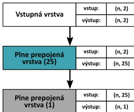
Obr. 4.2: Implementácia (hore) architektúry (dole) diskriminátora pre generovanie mocninovej funkcie x^2 . V pravej časti každého z troch blokov, ktoré znázorňujú jednotlivé vrstvy diskriminátora, je uvedený rozmer vstupných aj výstupných dát. Počet neurónov vrstvy je uvedený v zátvorke za jej názvom.
