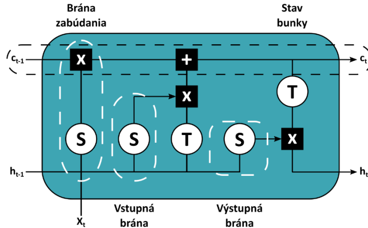
Obr. 1.14: Bunka LSTM a jej jednotlivé časti, prevzaté z [29]. Jedna LSTM bunka pozostáva zo 4 hlavných častí - stavom bunky (čierne prerušovaná čiara), a troch brán (biele prerušované čiary).
