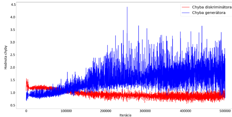
Obr. 5.7: Vývoj chýb diskriminátora a generátora počas učenia modelu GAN pre generovanie funkcie sínus s nemennou amplitúdou. Chyba diskriminátora bola počítaná ako súčet chýb diskriminátora na reálnych aj falošných dátach.
