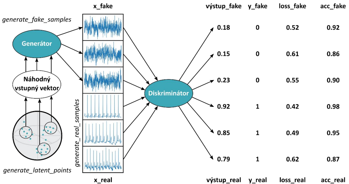
Obr. 4.20: Ukážka spôsobu osobitného trérovania diskriminátora na EKG signáloch. Všetky použité obrázky EKG signálov, sú z databázy signálov poskytnutých vedúcim tejto práce.
