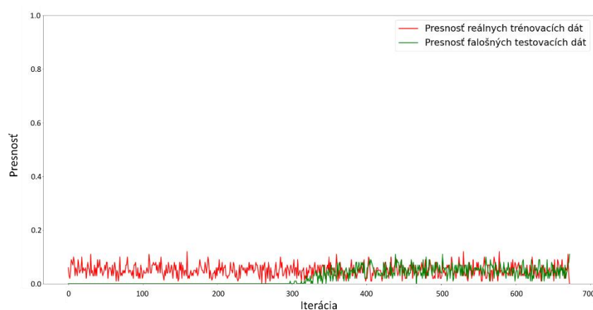
Obr. 5.18: Vývoj presností diskriminátoru na reálnych a falošných dátach počas tréningu modelu GAN pre generovanie EKG signálov.
