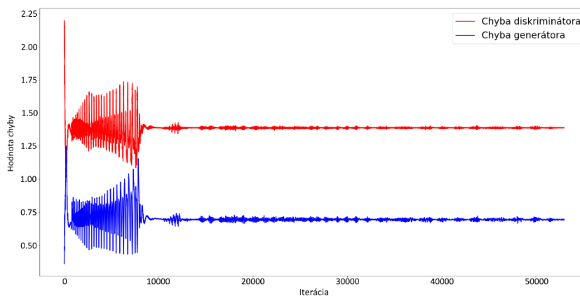
Obr. 5.3: Vývoj chýb diskriminátoru a generátoru počas učenia modelu GAN pre generovanie funkcie x^2 . Chyba diskriminátoru bola počítaná ako súčet chýb diskriminátoru na reálnych aj falošných dátach.
