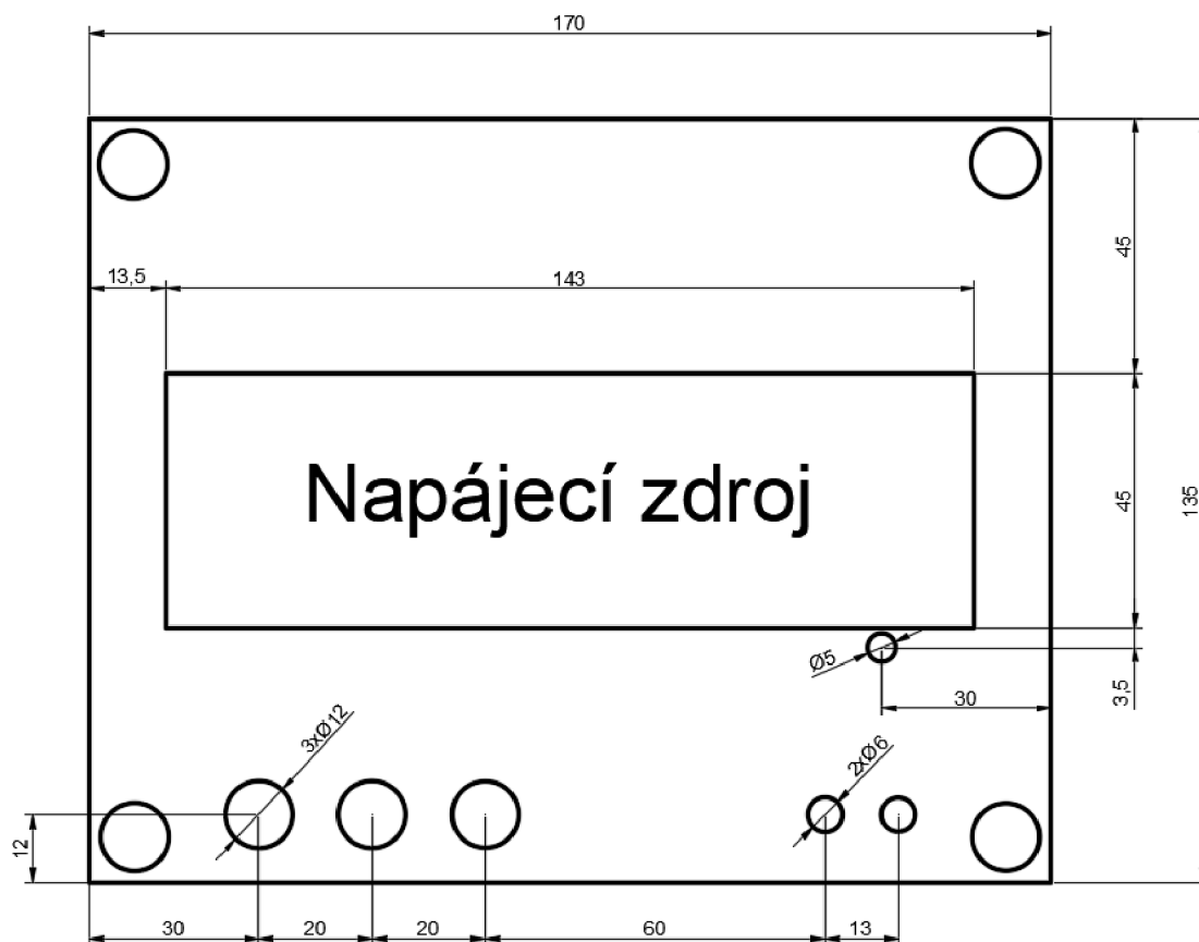
Obrázek 3.10 Šablona pro výrobu krabičky pro napájecí zdroj
