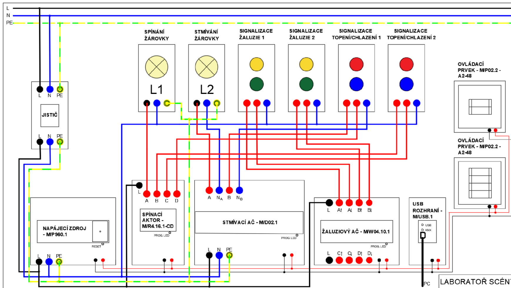
Obrázek 6.13 Schéma zapojení laboratorní úlohy
