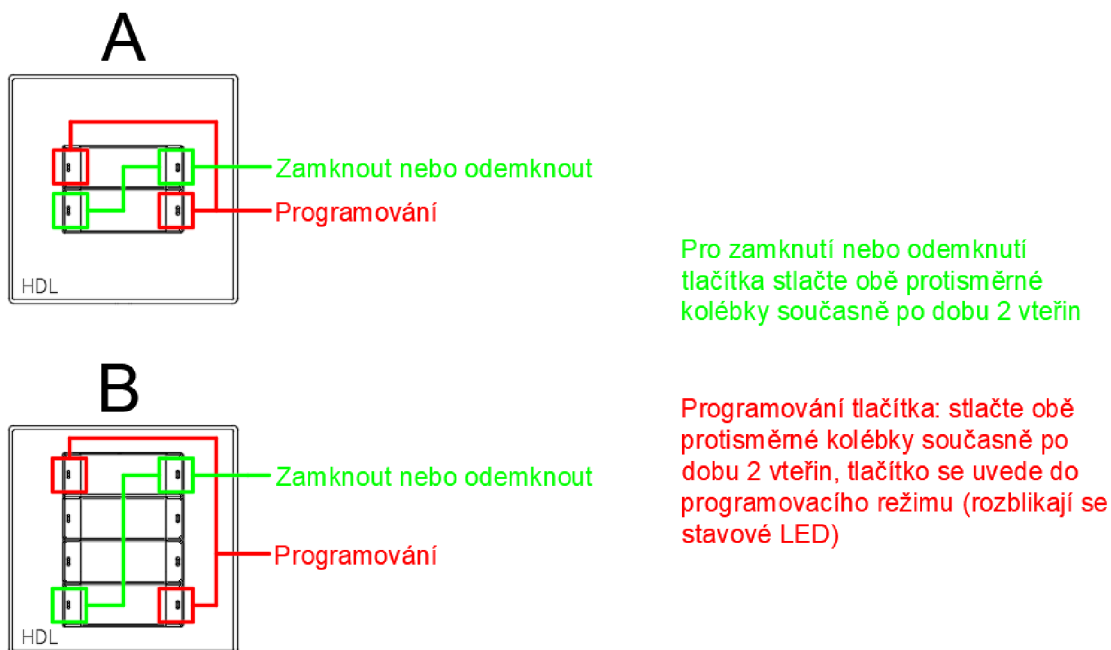
Obrázek 6.9 Programovací mód a zamykání HDL tlačítek
