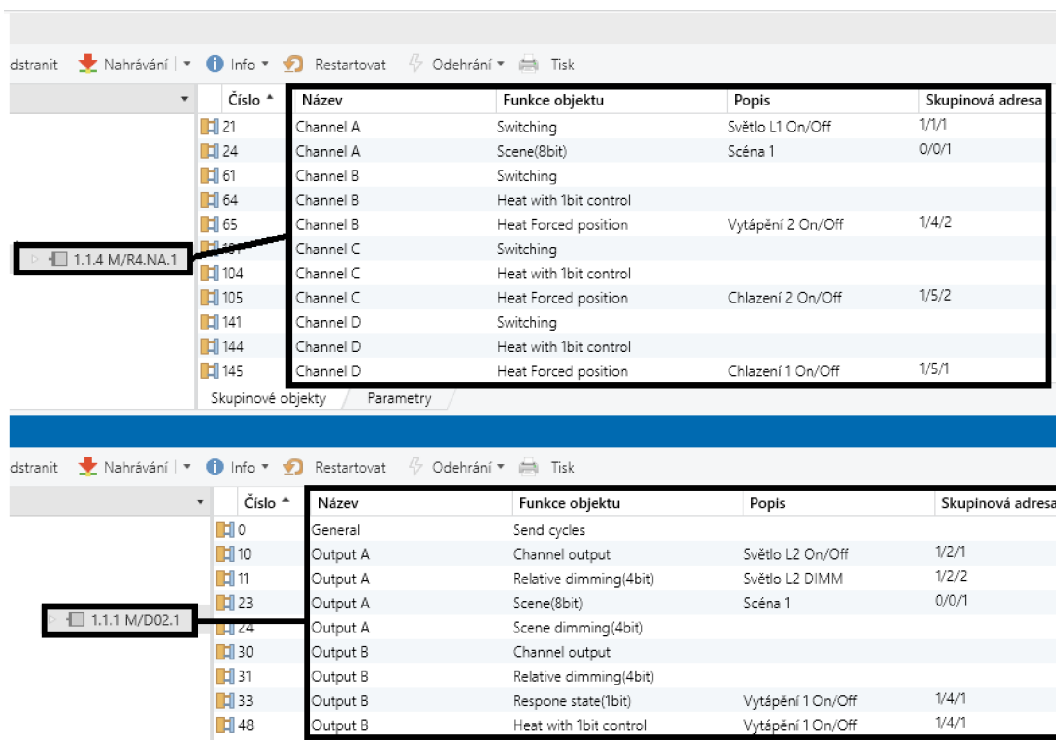
Obrázek 6.17 Přiřazení skupinových adres ke spínacímu a stmívacímu akтору
