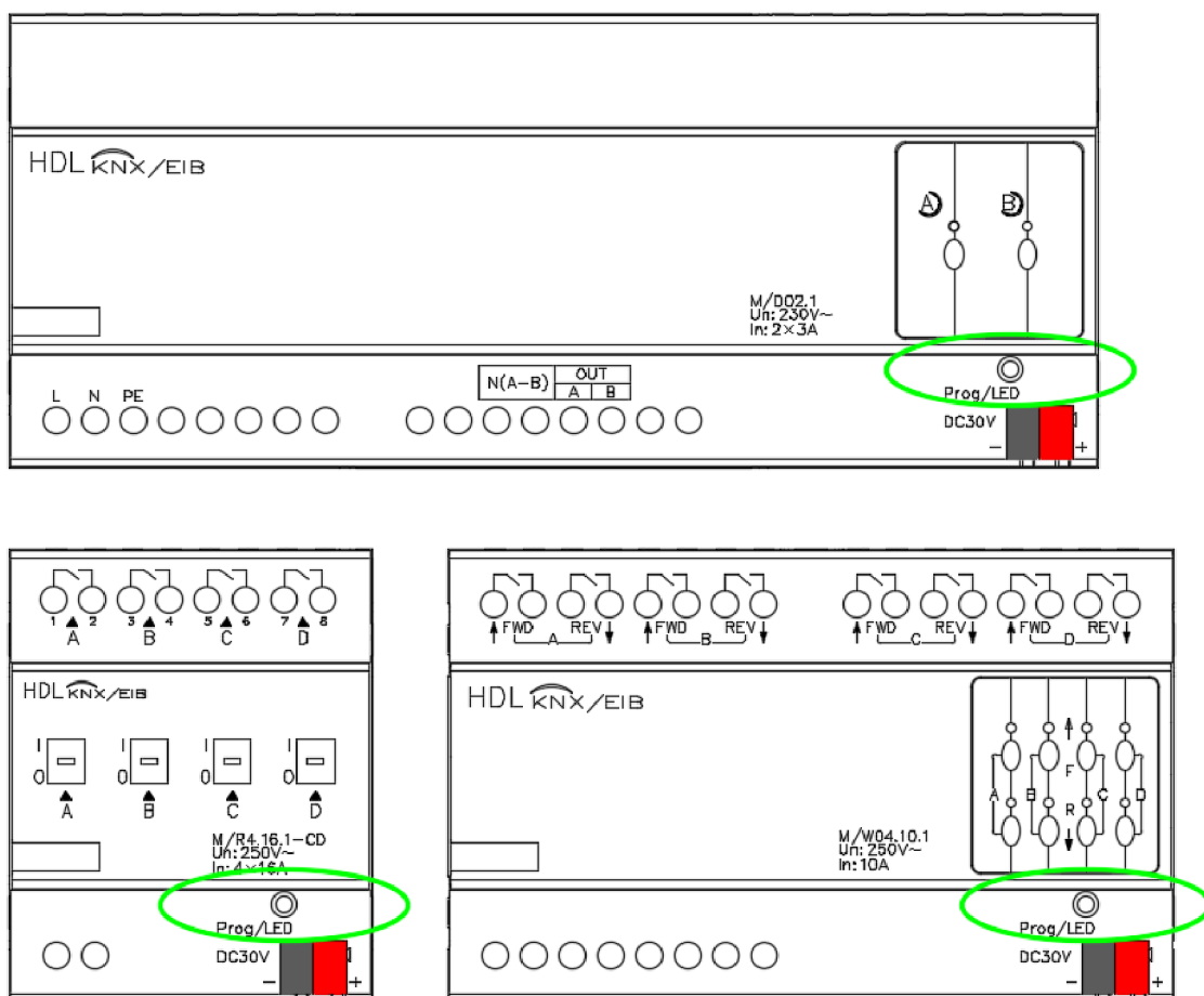
Obrázek 6.10 Programování akčních členů
