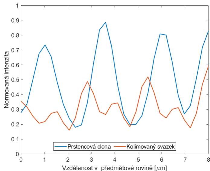
Obrázek 4.6: Porovnání sestavy s kolimovaným svazkem a sestavy s prstencovou clonou pro světelné pole. Vybraný 8. skupina a 2. element fázového USAF testu. Naznačení vybrané části na snímku 4.5.
