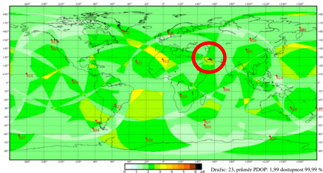
Obr. 24 Pokles dostupnosti GLONASS v 17:00 UTC (převzato z [82] a upraveno)
