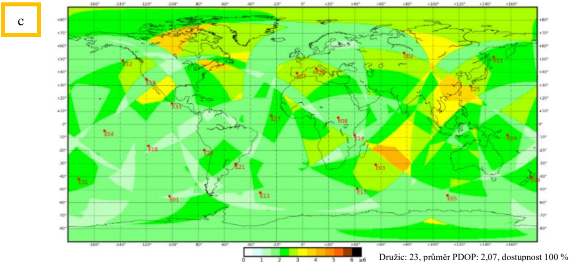
Obr. 23 PDOP pro GLONASS, GPS a Galileo v 09:00 UTC, dne 10.03.2021 (převzato z [82] a upraveno)
