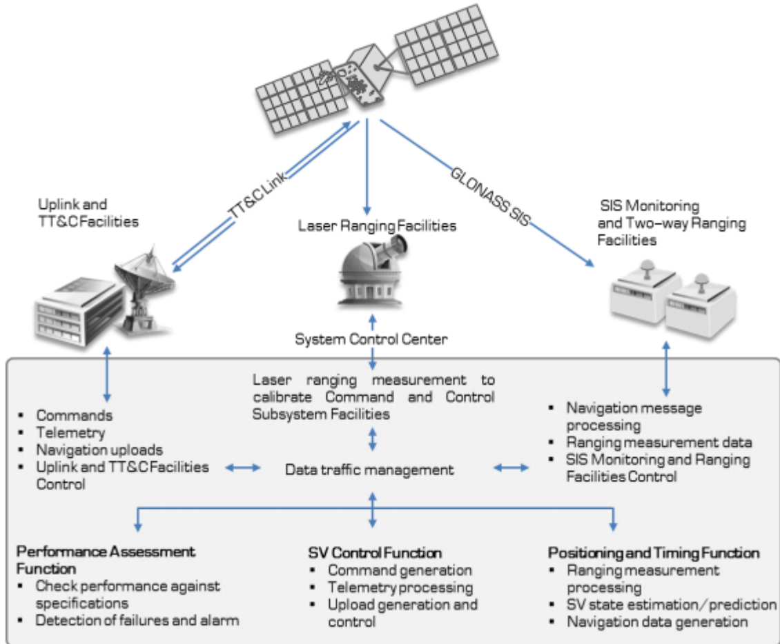
Příloha 5 Detailní přehled funkcí jednotlivých složek pozemního segmentu systému GLONASS (převzato z [86])
