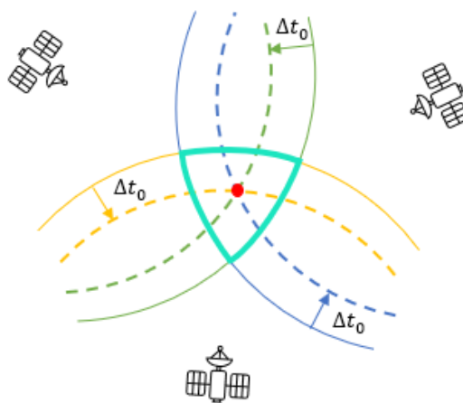
Obr. 6 Závislost časového posunu \Delta t_0 na poloze
