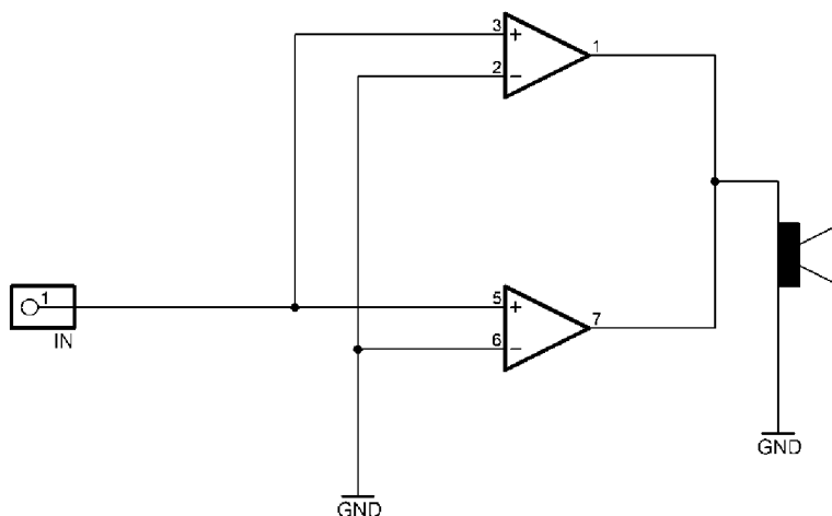
Obr. 17 Paralelní zapojení
