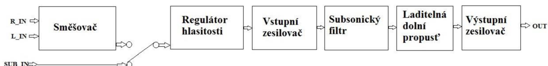
Obr. 9 Blokové schéma
