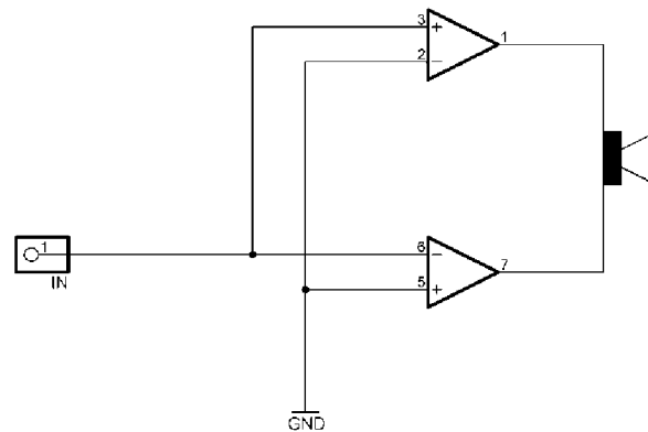
Obr. 16 Můstkové zapojení
