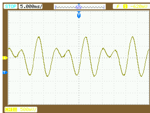
Obr. 21 Záznam směšovače z osciloskopu
