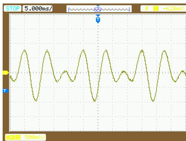
Obr. 22 Záznam směšovače s funkcí otočení fáze
