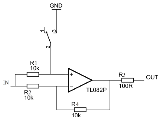
Obr. 15 Schéma výstupního zesilovače
