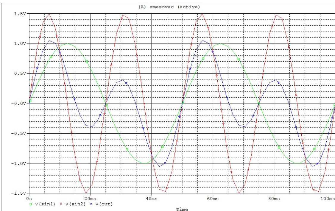
Obr. 12 Časová charakteristika směšovače s rozdílnými vstupy
