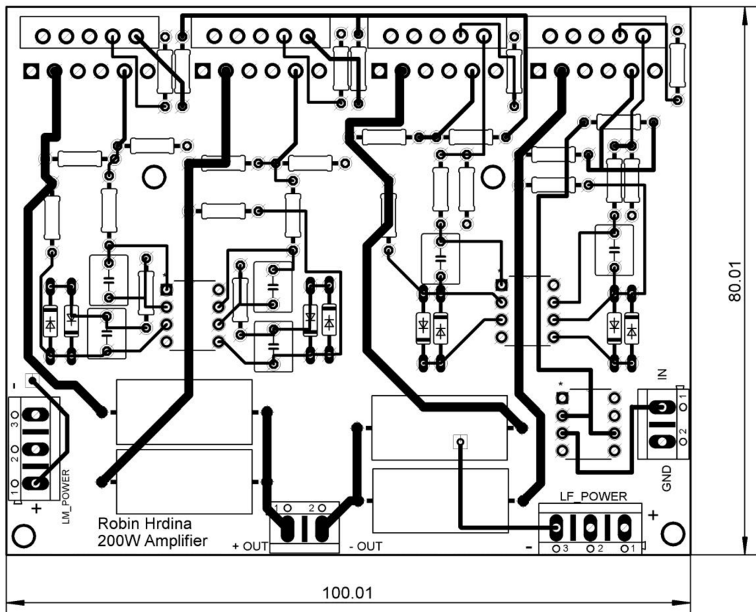
Obr. 30 Strana TOP koncového stupněň
