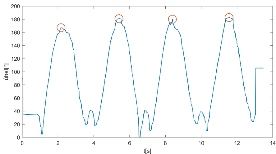
Obr. 6.2: Vykreslení výpočtu úhlu při VF v rozsahu pohybu 0-180°, maxima znázorněna funkcí findpeaks
