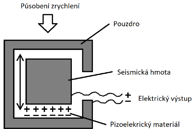
Obr. 2.1: Základní schéma piezoelektrického senzoru
