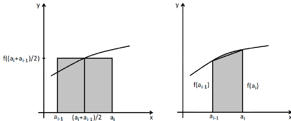
Obr. 3.4: Porovnání dvou integračních metod: obdelníkové (vlevo) a lichoběžníkové (vpravo)
