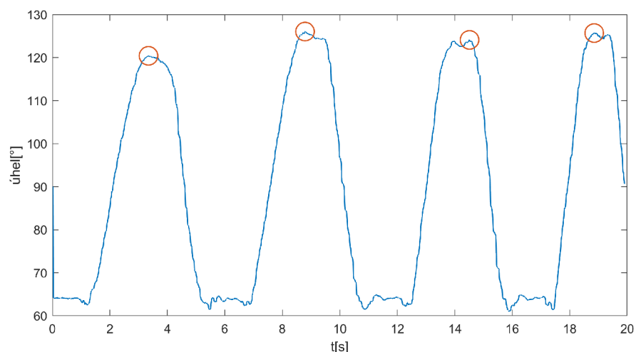
Obr. 6.3: Vykreslení výpočtu úhlu při abdukci v rozsahu pohybu 0-180°, maxima znázorněna funkcí findpeaks
