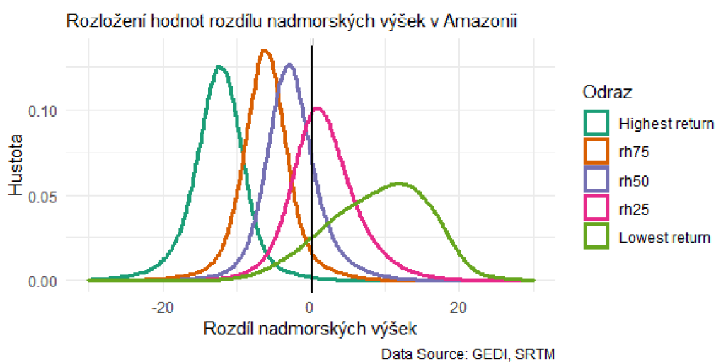
Obrázek 16: Density plot rozdílu nadmořských výšek v Amazonii (GEDI, SRTM)
