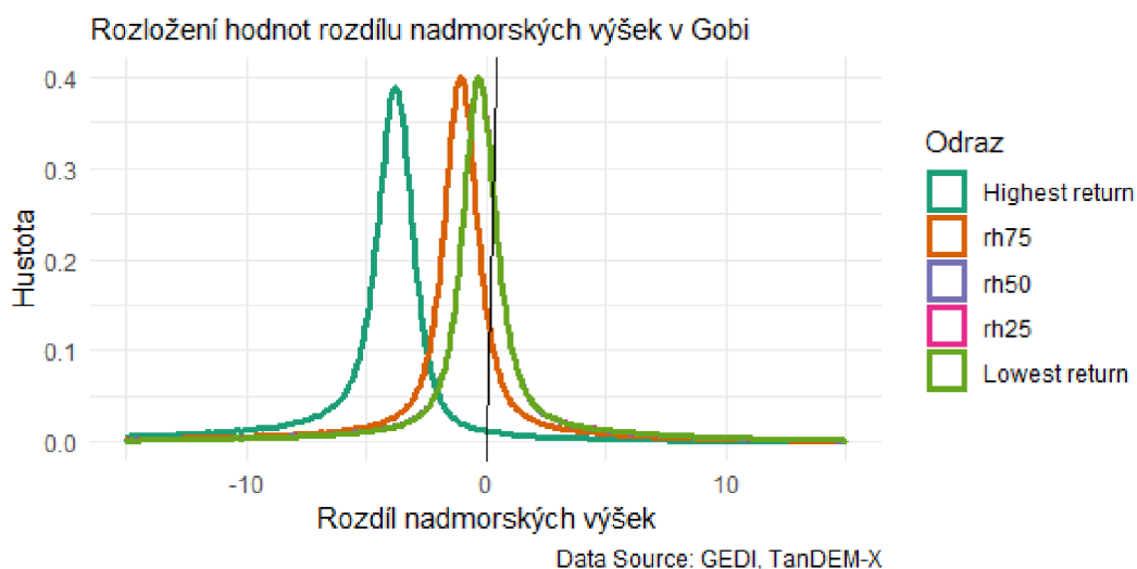
Obrázek 17: Density plot rozdílů nadmorských výšek v poušti Gobi (GEDI, TDX)
