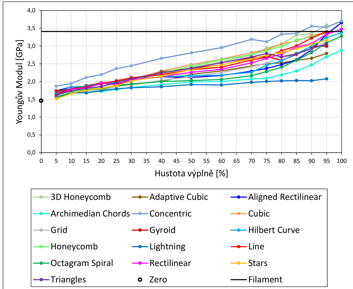
Obr. 50 Hodnoty Youngova modulu pro všechny testované varianty a samotný filament
