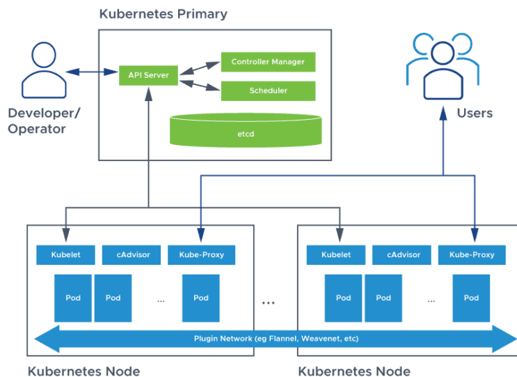
Obrázek 3 Architektura Kubernetes [13]
