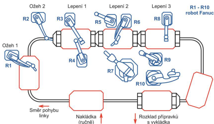
Obr. 37 Schéma lepicí linky
