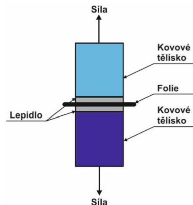
Obr. 15 Schéma tahové zkoušky lepeného spoje [17]
