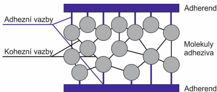
Obr. 4 Lepený spoj [17]
