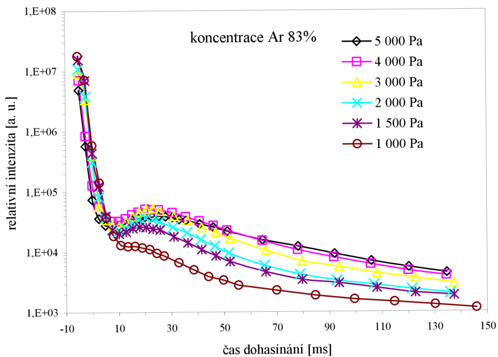
Obr. 11: Průběh intenzity pásu 2-0 prvního pozitivního systému dusíku, koncentrace argonu 83 %, různé tlaky.
