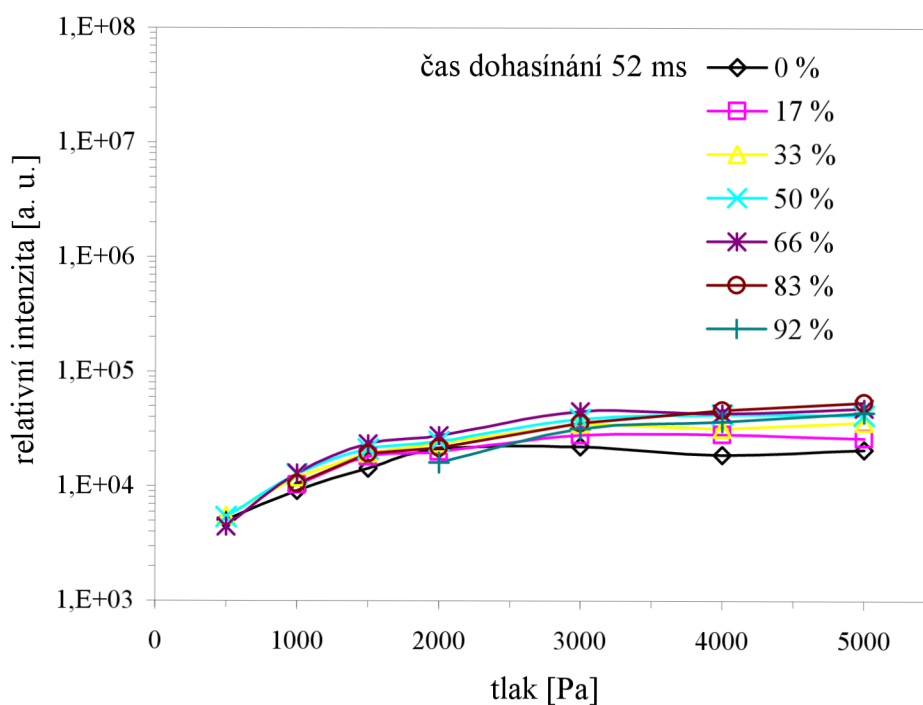
Obr. 20: Závislost intenzity pásu 11-7 prvního pozitivního systému dusíku na tlaku pro různé koncentrace argonu v čase dohasínání 52 ms.
