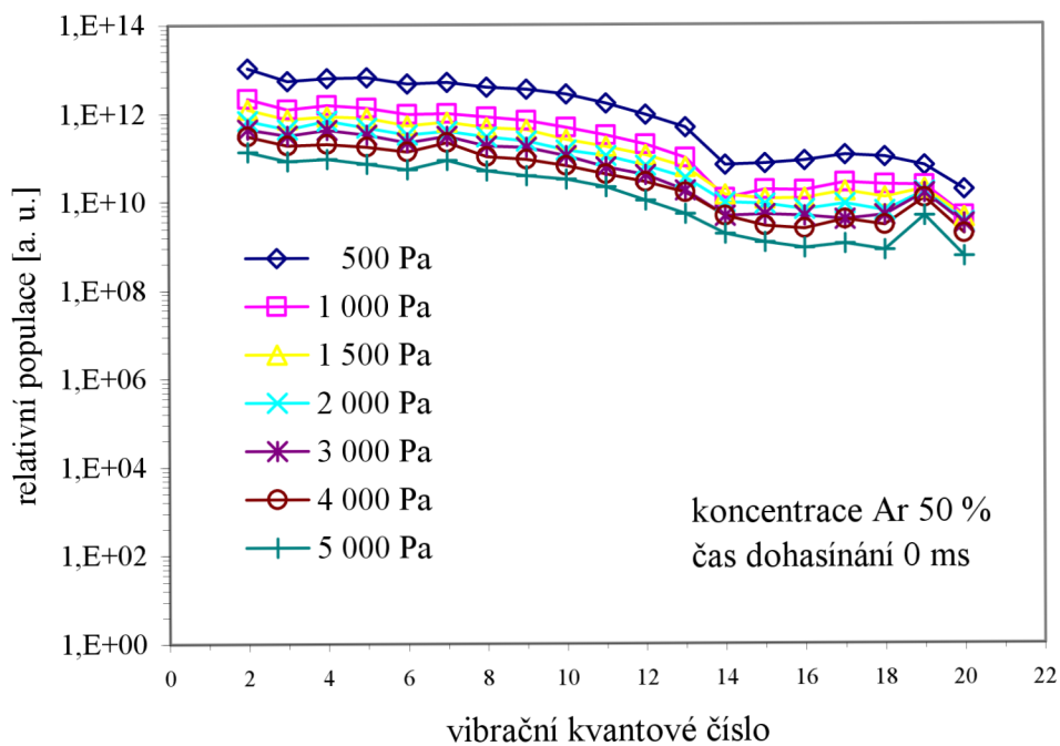
Obr. 22: Vibrační rozdělení stavu N_2(B^3\Pi_g) pro koncentraci argonu 50 % v čase dohasinání 0 ms.
