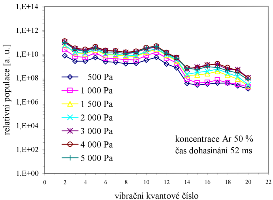
Obr. 24: Vibrační rozdělení stavu N_2(B^3\Pi_g) pro koncentraci argonu 50 % v čase dohasinání 52 ms.
