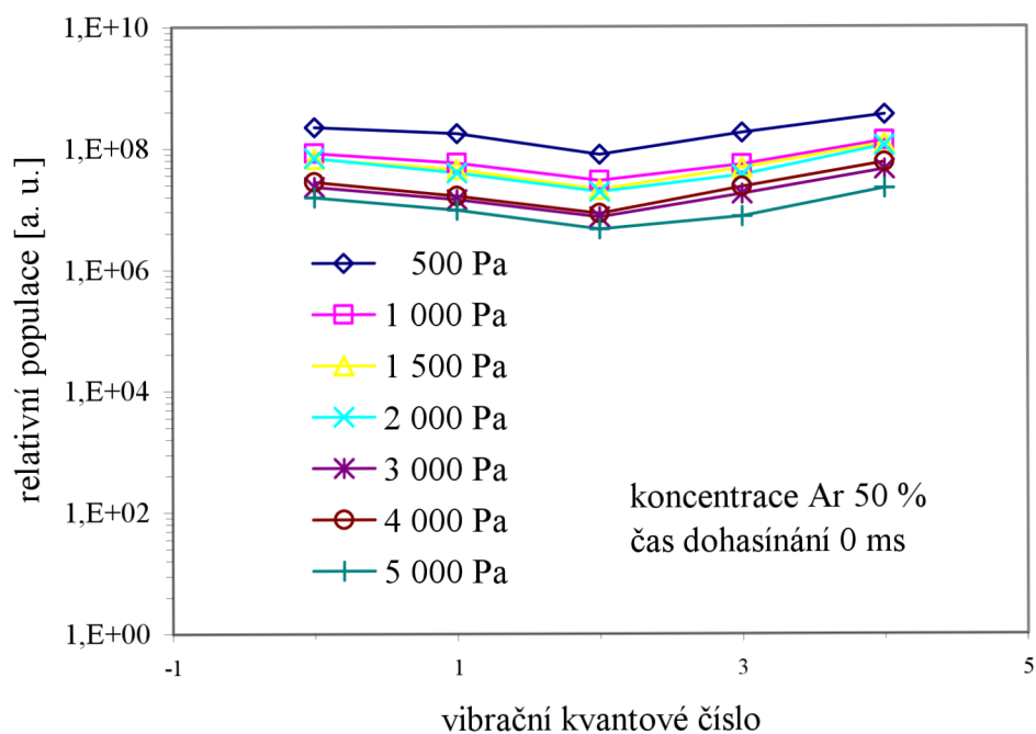
Obr. 30: Vibrační rozdělení stavu N_2 (C^3\Pi_u) pro koncentraci argonu 50 % v čase dohasinání 0 ms.
