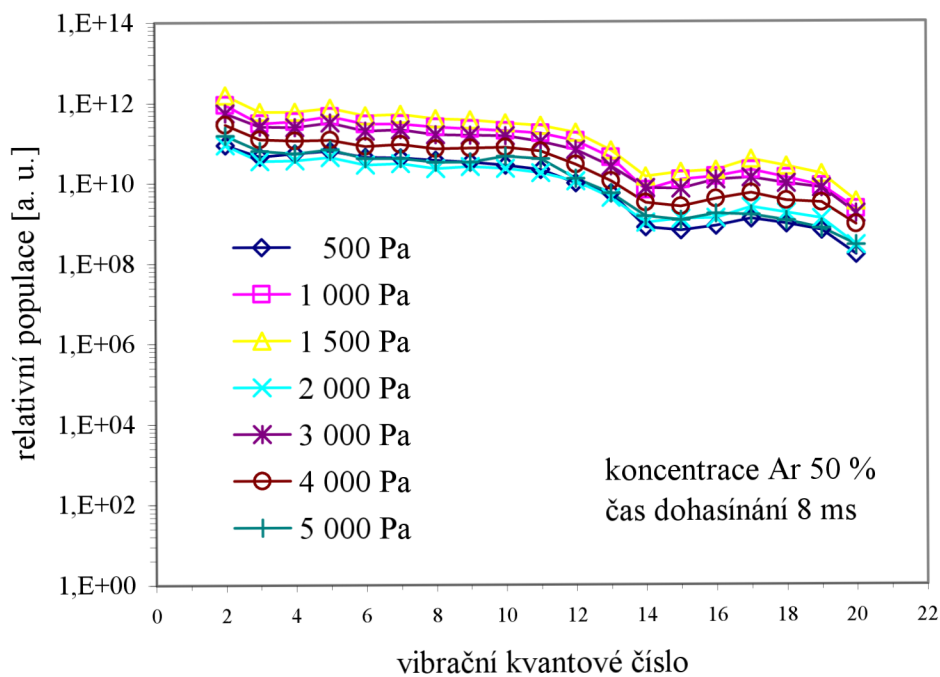
Obr. 23: Vibrační rozdělení stavu N_2(B^3\Pi_g) pro koncentraci argonu 50 % v čase dohasinání 8 ms.
