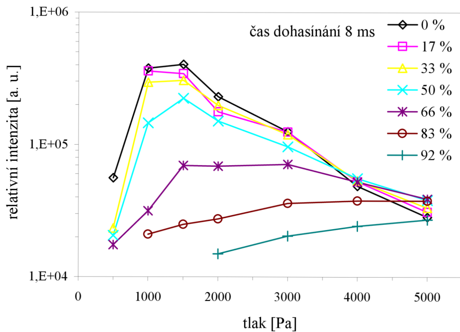
Obr. 19: Závislost intenzity pásu 11-7 prvního pozitivního systému dusíku na tlaku pro různé koncentrace argonu v čase dohasínání 8 ms.
