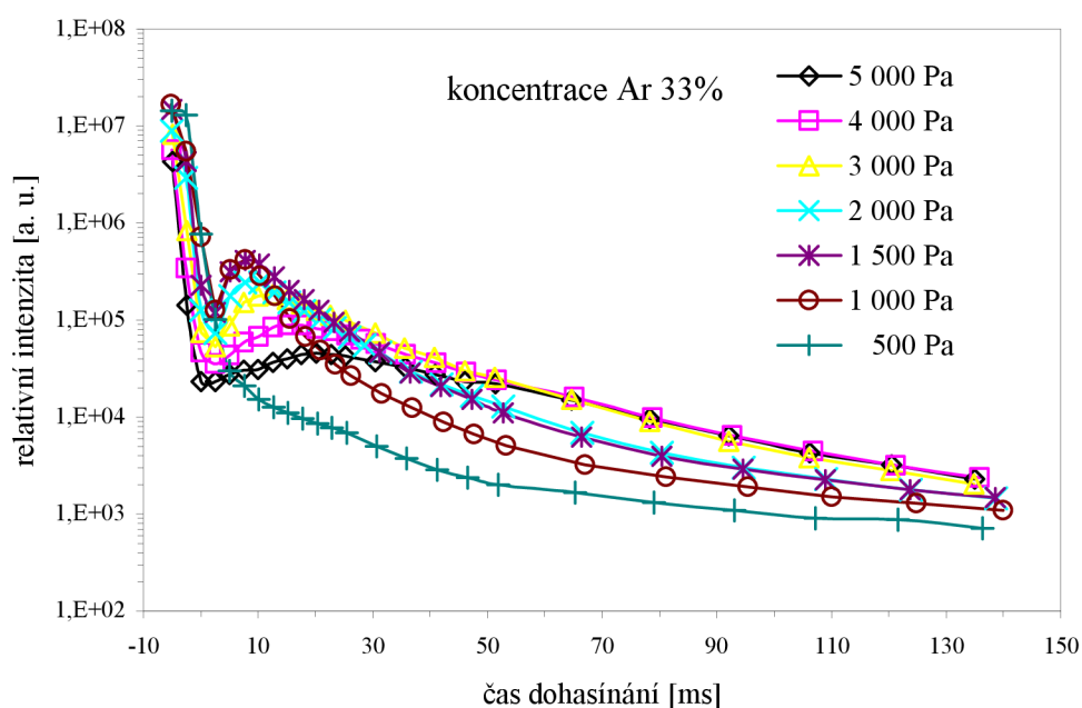
Obr. 9: Průběh intenzity pásu 2-0 prvního pozitivního systému dusíku, koncentrace argonu 33 %, různé tlaky.
