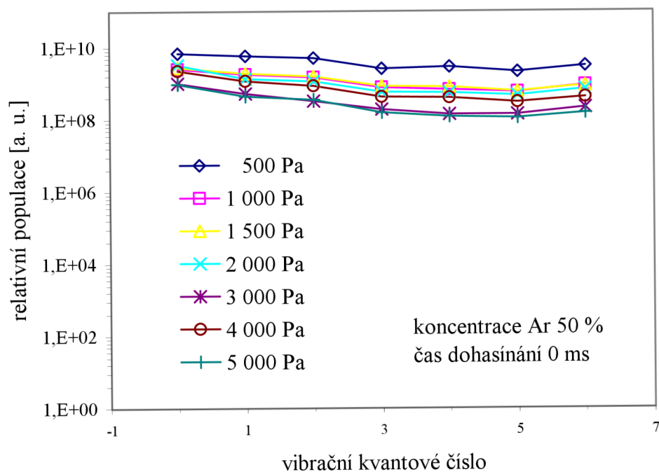
Obr. 26: Vibrační rozdělení stavu N_2^+ (B^2\Sigma_u^+) pro koncentraci argonu 50 % v čase dohasinání 0 ms.
