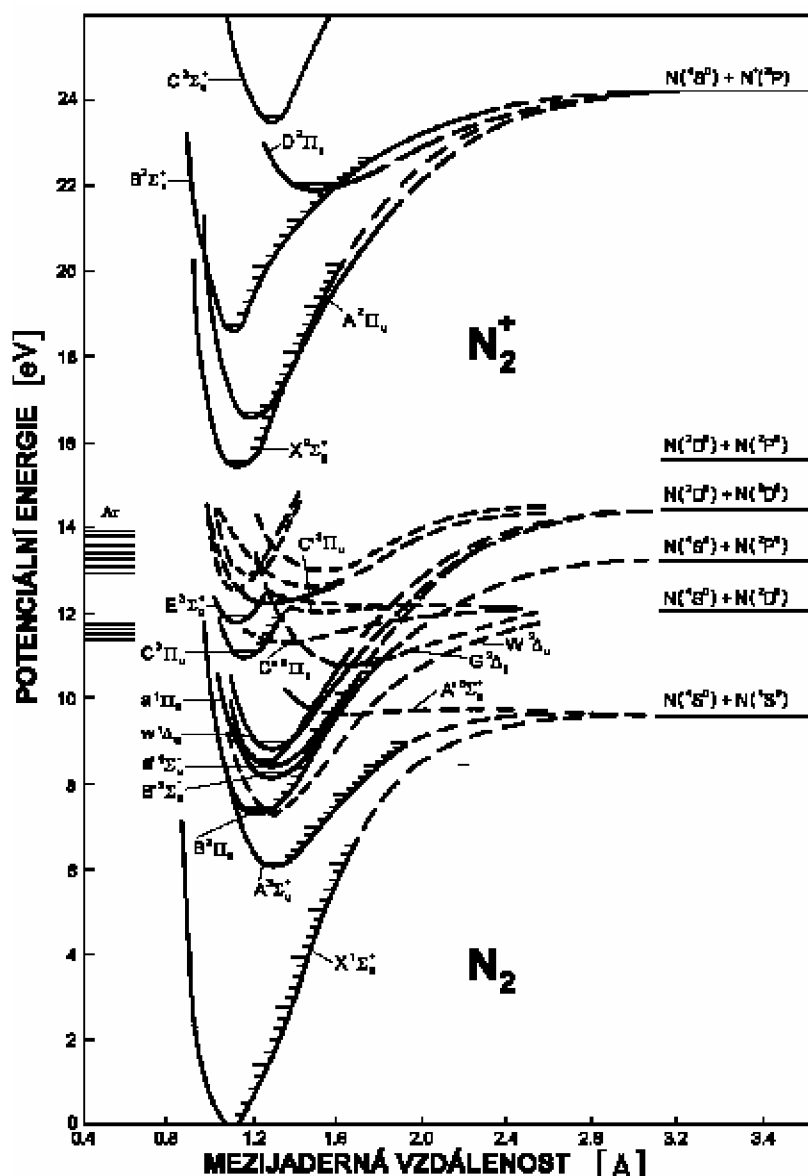
Obr. 3: Energetické schéma molekuly dusíku [27] s naznačenými hladinami argonu [28], detailní popis hladin argonu lze nalézt v databázi (viz. seznam použitých zdrojů) [28].
