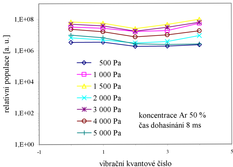
Obr. 31: Vibrační rozdělení stavu N_2 (C^3\Pi_u) pro koncentraci argonu 50 % v čase dohasinání 8 ms.
