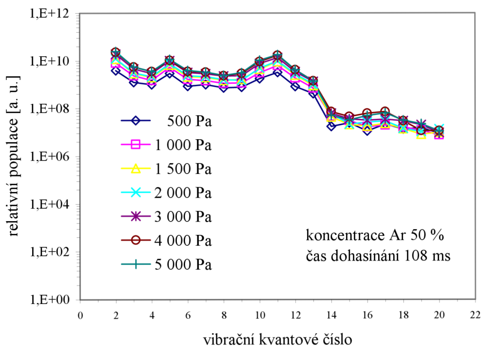
Obr. 25: Vibrační rozdělení stavu N_2(B^3\Pi_g) pro koncentraci argonu 50 % v čase dohasinání 108 ms.
