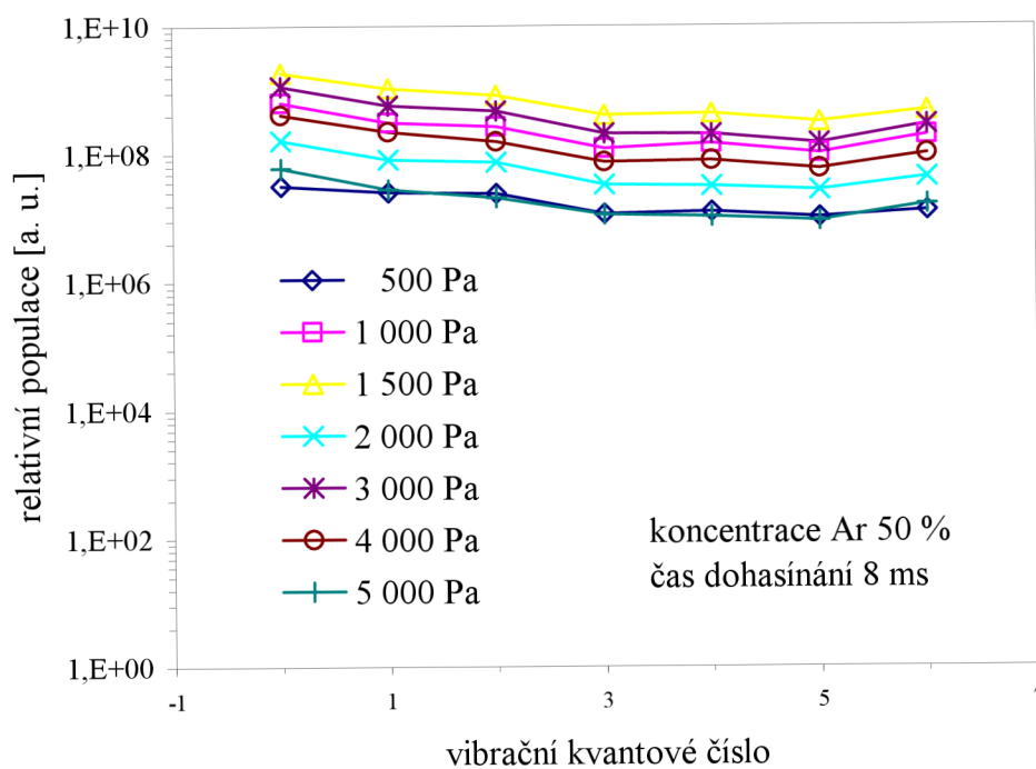
Obr. 27: Vibrační rozdělení stavu N_2^+ (B^2\Sigma_u^+) pro koncentraci argonu 50 % v čase dohasinání 8 ms.
