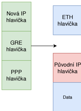
Obrázek 4.6: Paket obsahující PPTP zapouzdření
