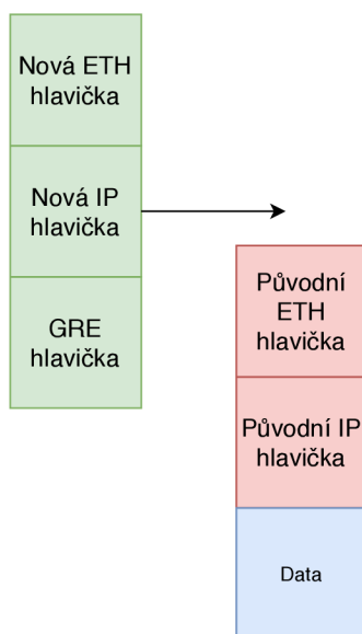
Obrázek 4.4: Paket obsahující GRE TAP zapouzdření
