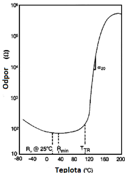
Obrázek 6: Teplotní závislost PTC termistoru, převzatá z [19]
