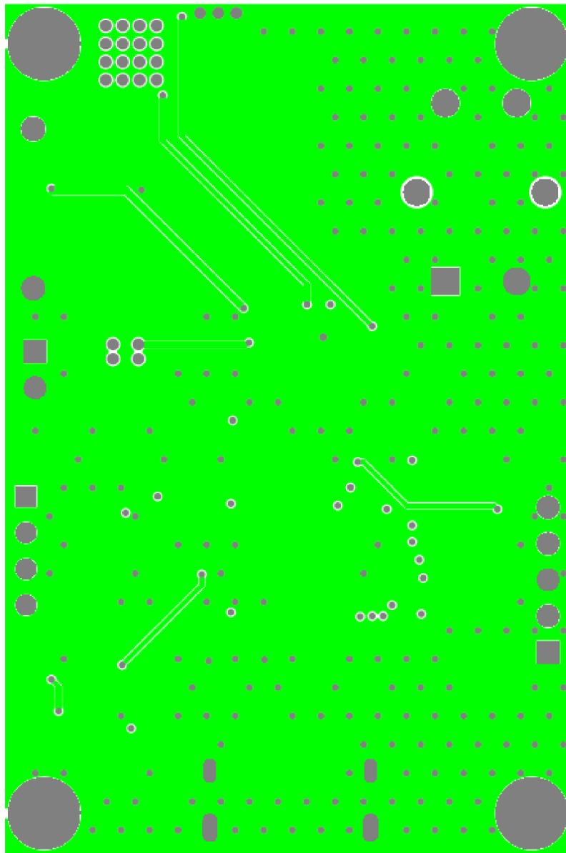
Obrázek A 4: Vnitřní vrstva signálová
