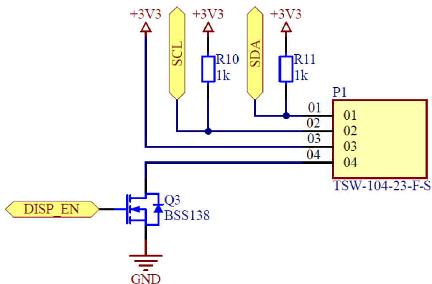
Obrázek 19: Schéma zapojení k modulu SSD1306
