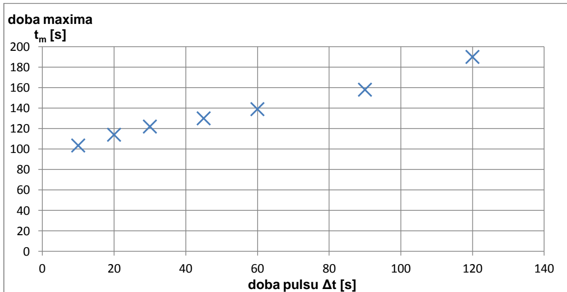
Graf č. 16: Pórobeton Ytong, U_z = 11 \text{ V} , r = 1,3 \text{ cm} , termistor, \Delta t = 10 až 120 \text{ s} – doba teplotního maxima
