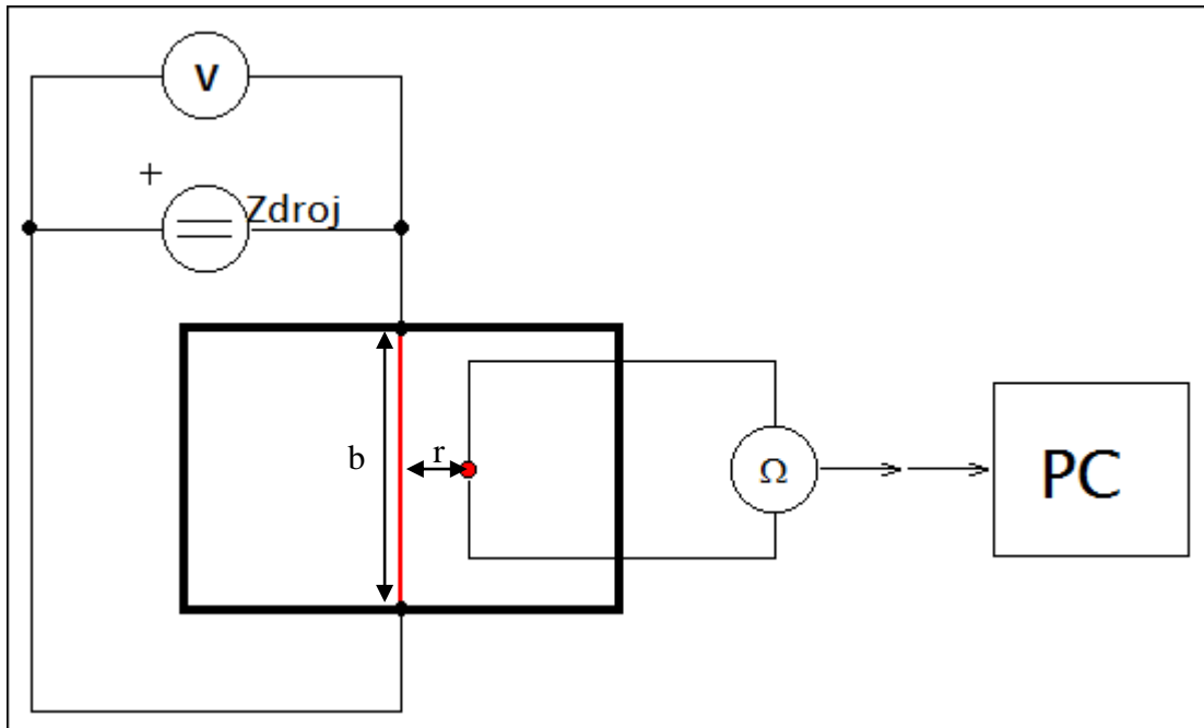
Obrázek č. 1: Schéma měřícího přípravku s lineovým zdrojem
