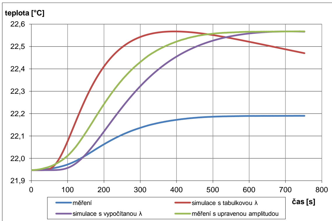
Graf č.4: Pálená cihla, I = 5 \text{ A} , U = 1,459 \text{ V} , \Delta t = 60 \text{ s} , termistor
