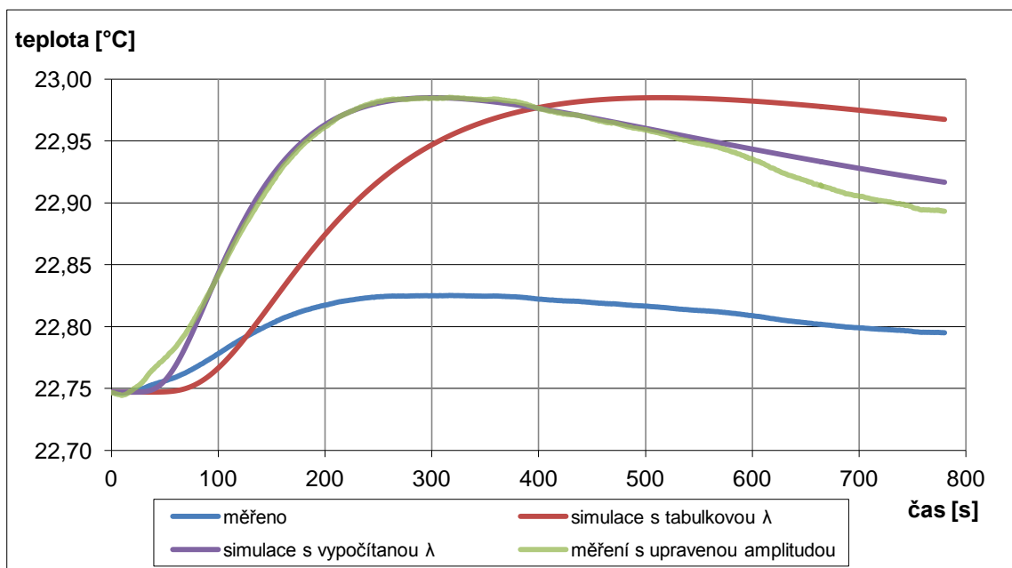
Graf č. 2: Vápenopísková cihla, I = 5 \text{ A} , U = 1,52 \text{ V} , \Delta t = 30 \text{ s} , termistor
