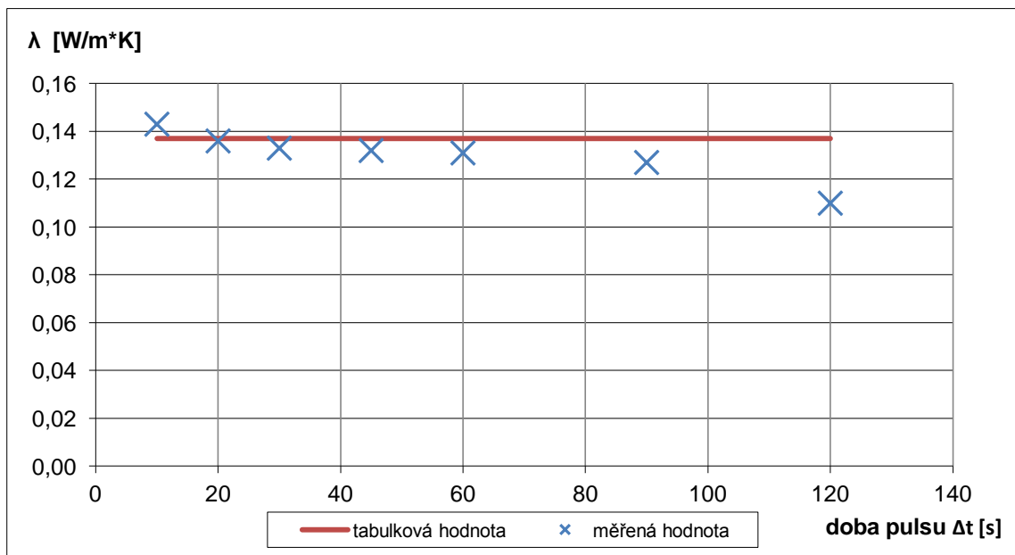
Graf č. 17: Pórobeton Ytong, U_z = 11 \text{ V} , r = 1,3 \text{ cm} , termistor, \Delta t = 10 až 120 \text{ s} – tepelná vodivost
