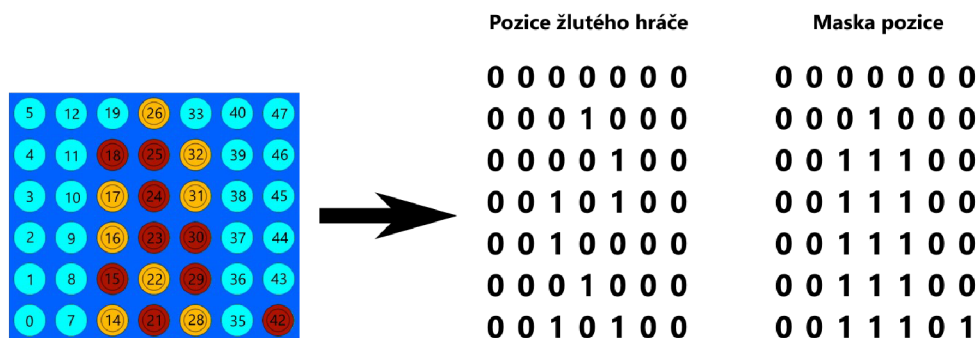
Obrázek 31: Zakódování herní pozice
