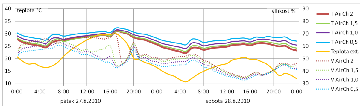
Obr.12 Začátek víkendových dnů - průběhy teploty vzduchu a relativní vlhkosti při různých okrajových podmínkách (různé intenzitě větrání) v obývacím pokoji ve dnech 27.-28.8. 2010.
