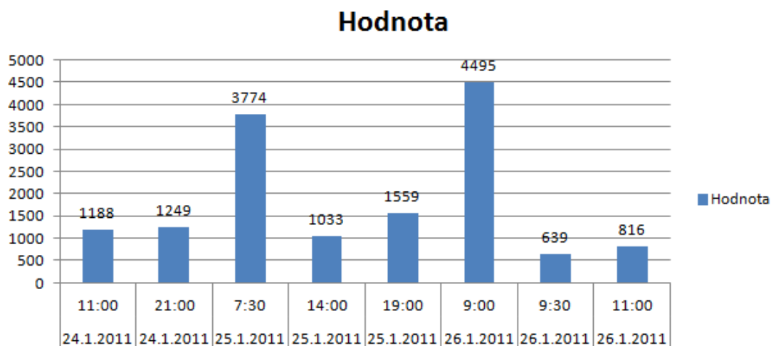
Obr.8 Měřené hodnoty koncentrace CO 2 v RD2
