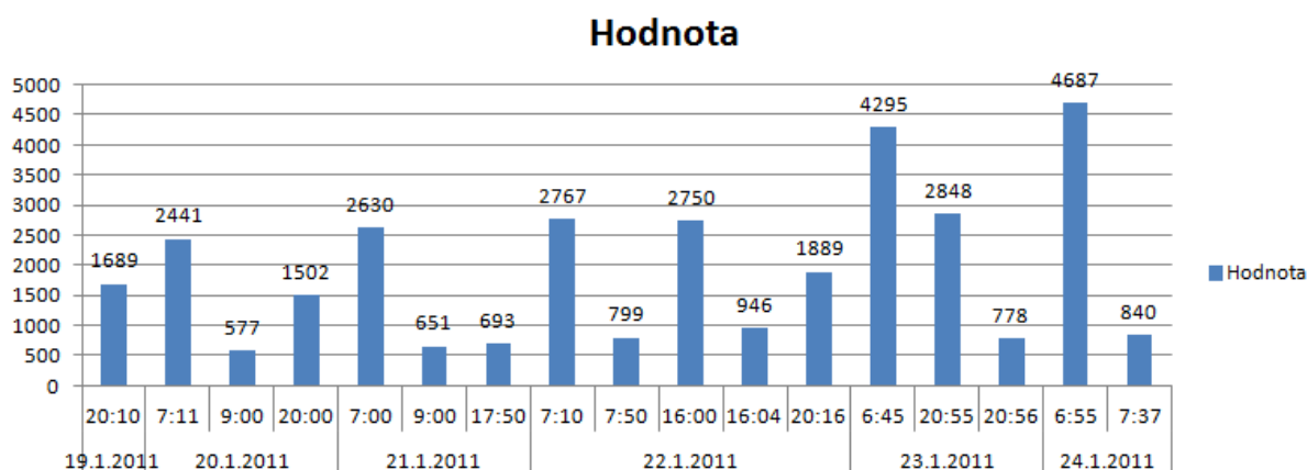
Obr. 7 Měřené hodnoty koncentrace CO 2 v RD1
