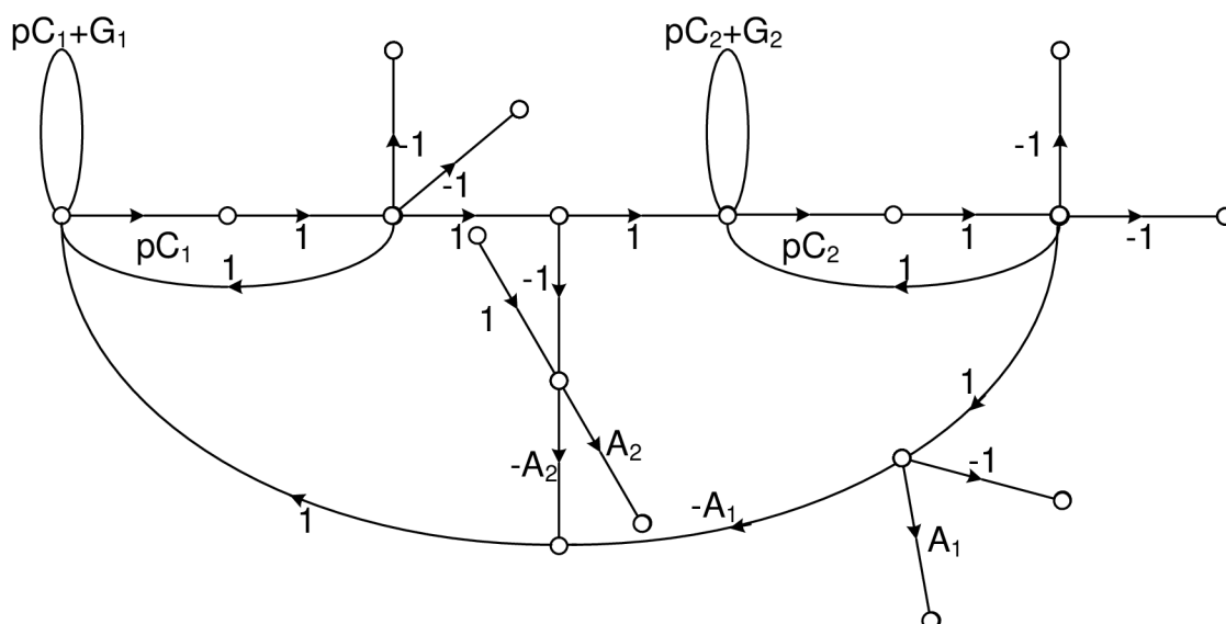
Obr.5.21: M-C graf navrženého plně diferenčního univerzálního kmitočtového filtru se dvěma říditelnými DACA prvky
