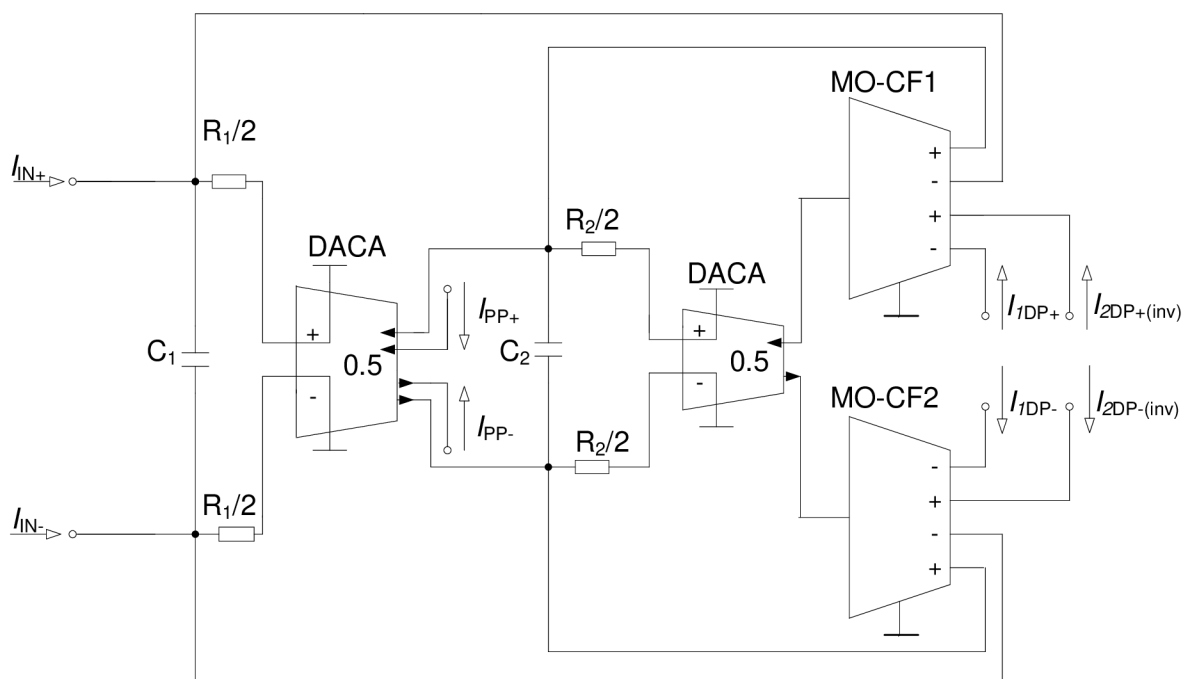
Obr.6.5: Schéma zapojení navrženého plně diferencního filtru
