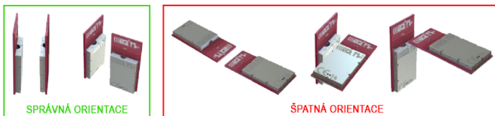
Obrázek 3.5: Orientace Transceiveru [52]
