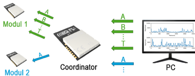
Obrázek 4.14: Znázornění zvoleného způsobu vyčítání dat
