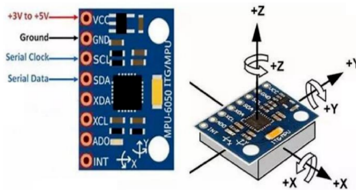
Obrázek 3.2: Akcelerometr GY-521 [49]
