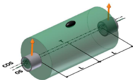
Obrázek 1.6: Statická nevyváženost [1]
