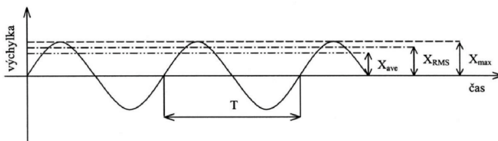
Obrázek 1.2: Parametry signálu[1]
