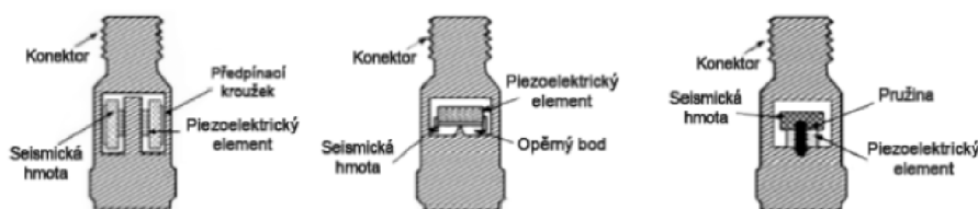
Obrázek 1.15: Provedení piezoelektrických akcelerometrů [15]
