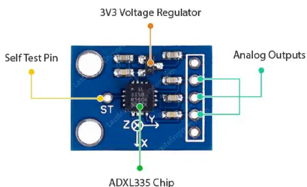
Obrázek 3.3: Akcelerometr ADXL335 [50]
