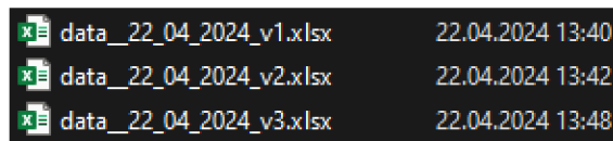
Obrázek 4.8: Výstupní soubory
