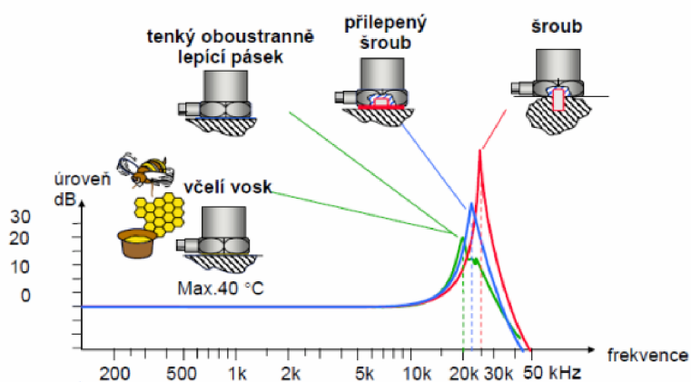
Obrázek 1.18: Uchycení snímačů[13]
