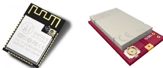
Obrázek 5.2: ESP32-S a TR-72D, vybavené konektory U.FL
