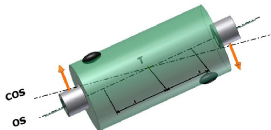
Obrázek 1.7: Momentová nevyváženost [1]
