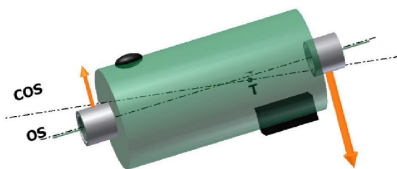
Obrázek 1.8: Dynamická nevyváženost [1]
