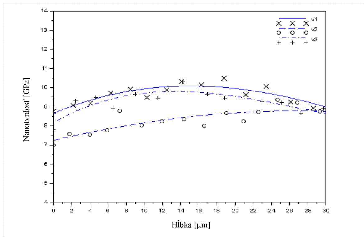
Obr. 25 Nanotvrdosti vzoriek.
