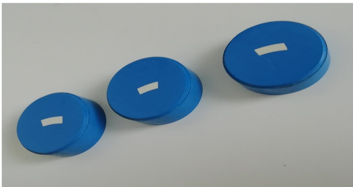
Obr. 9 Metalografické vzorky.
