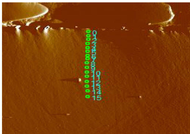
Naznačenie vpichov nanointendora pri vzorke číslo 1.
