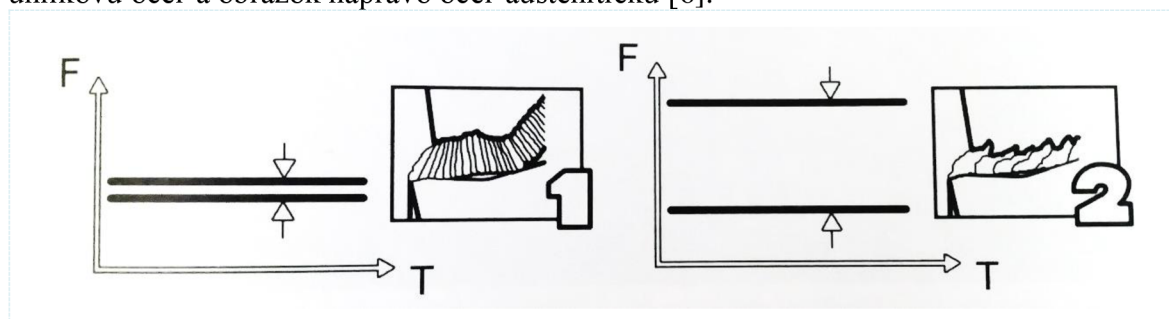
Obr. 5 Rozdiel vo výkyvoch reznej sily [6].
