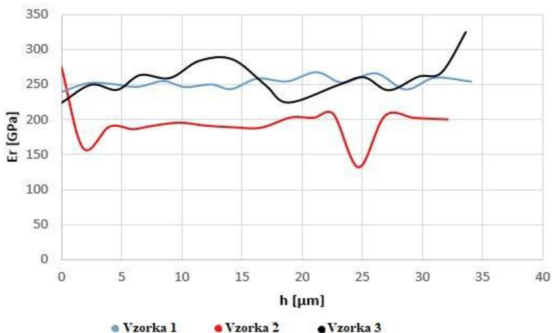
Obr. 23 Vpichy nanoindentora.
