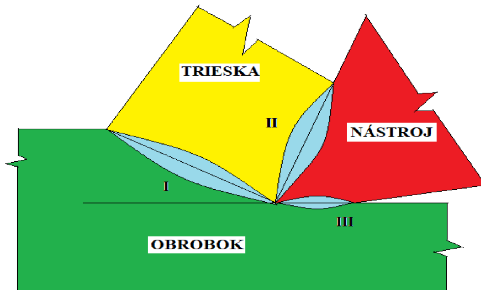
Obr. 4 Deformačné zóny – podľa [12]
