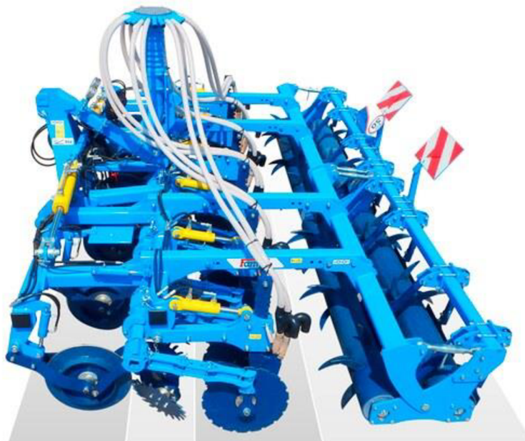
Obrázek 14 Farmet pásový kypřič strip-till (Farmet s.r.o.)
