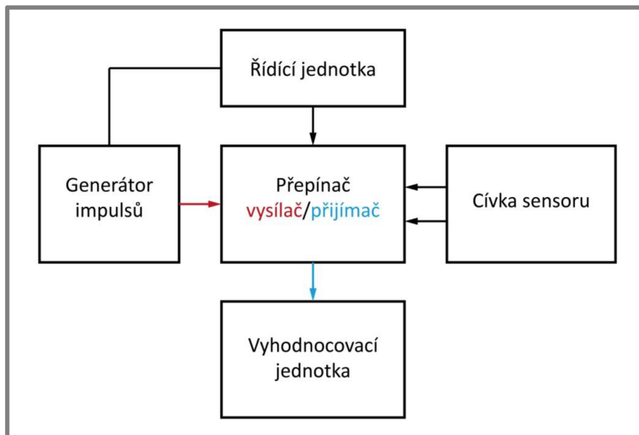
Obr. 2-12 Schéma pulzní indukce [2]
