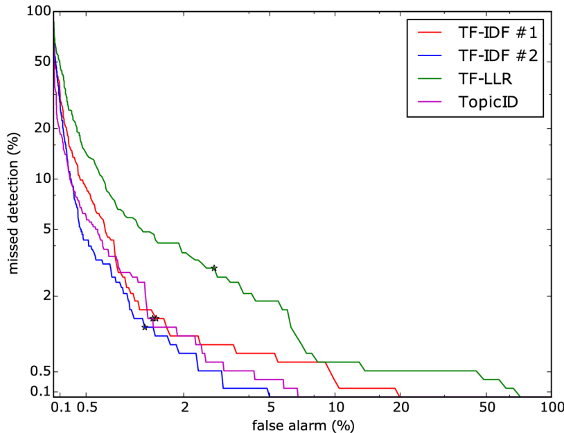
Obrázek 5.2: DET křivka ukazující závislost missed detection a false alarm na posunujícím se prahu. Hodnoty jsou ukládány po 0.001 (posunující se práh). Čím blíže je křivka k osám, tím je její úspěšnost lepší. Dále má každá z křivek bod, který je označován EER - equal error rate (hvězdička), který označuje místo, kde si jsou obě hodnoty nejpodobnější (a zároveň nejnižší). Čím bude tento bod blíže k 0, tím lépe budou hodnoty porovnání článků stejných a jiných témat separované.
