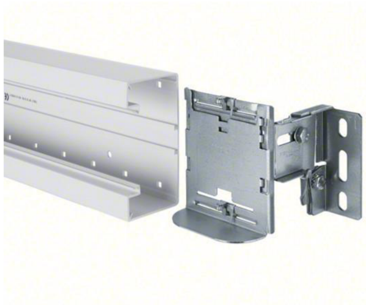
Obrázek 20:tehalit.BRHP parapetní kanál PC/ABS, bezhalogenový (Zdroj: [19])
