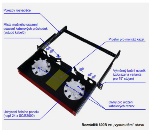
Obrázek 30: Optický rozváděč 600
