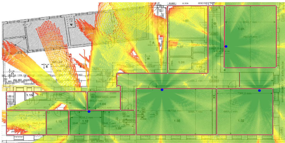
Obrázek 10: Pokrytí signálem 2,4 GHz
