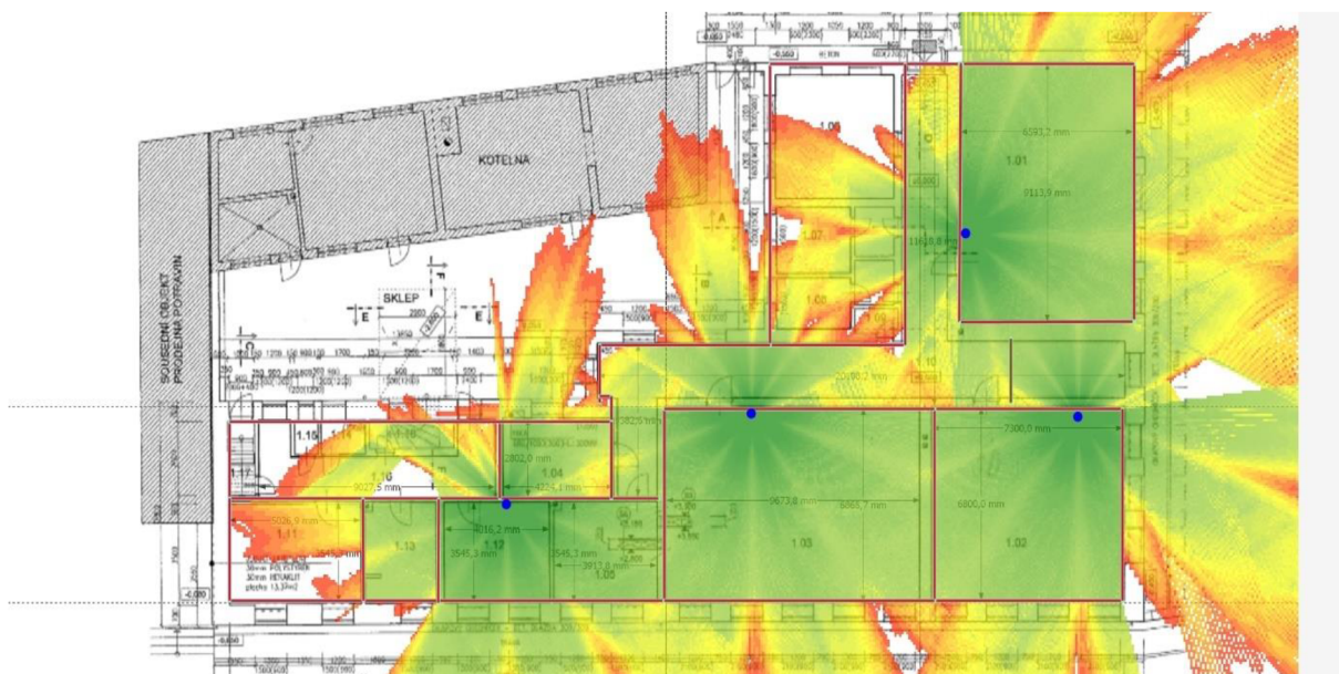
Obrázek 11: Pokrytí signálem 5 GHz
