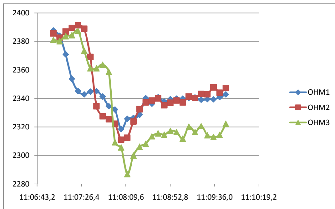
Obrázek 15 Průběh naměřených funkcí závislosti odporu termistoru na teplotě
