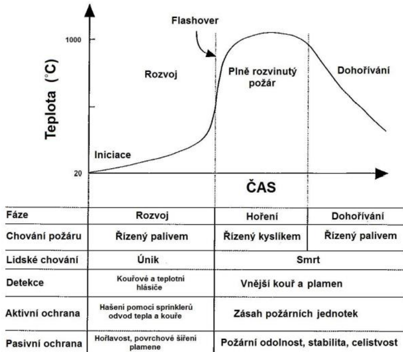
Obr.1 Význam fází požáru z hlediska požární bezpečnosti dřevostaveb [1]
