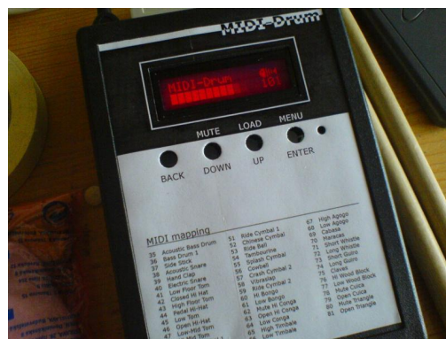
Obrázek 2.4: Zapojený prototyp MIDI-Drum, bez tlačítek.
