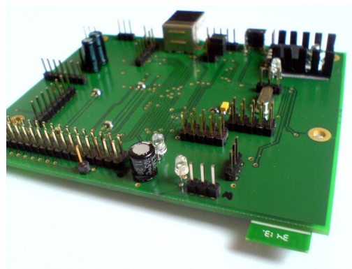
Obrázek 5.2: Osazená hlavní deska, strana součástek.
