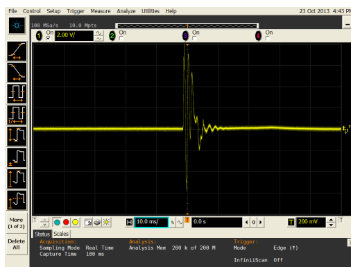
Obrázek 3.2: Průběh napětí na piezoměničích při úderu, časová osa 10 ms / div.
