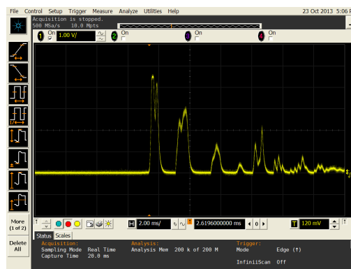
Obrázek 3.3: Průběh napětí na výstupu desky zesilovače, časová osa 2 ms / div.
