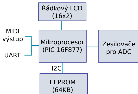
Obrázek 2.3: Blokové schéma prototypu MIDI-Drum.
