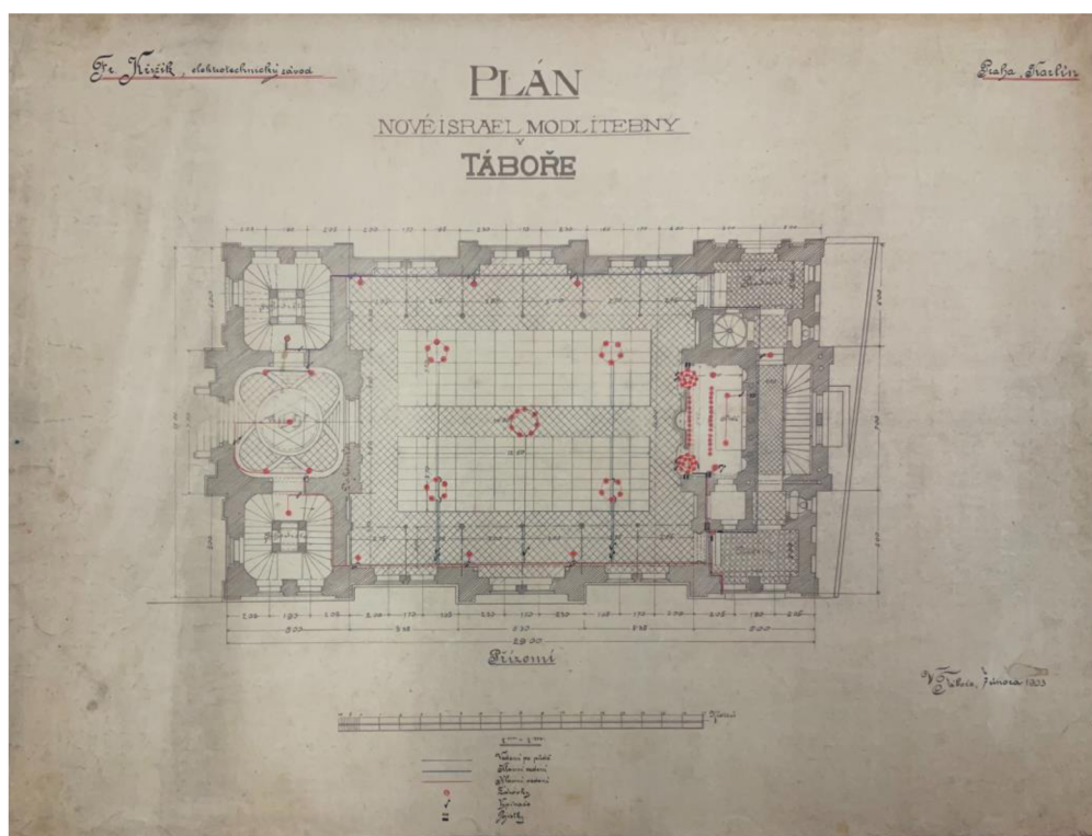
[12] Stavební náčrt synagogy, 1883, Josef V. Staněk.
