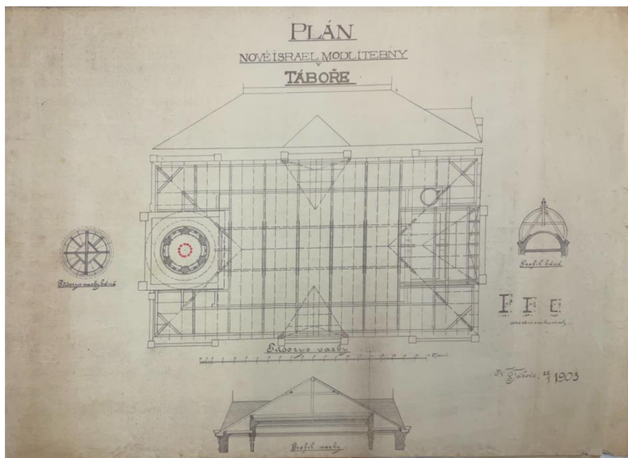
[11] Stavební náčrt synagogy, 1883, Josef V. Staněk.
