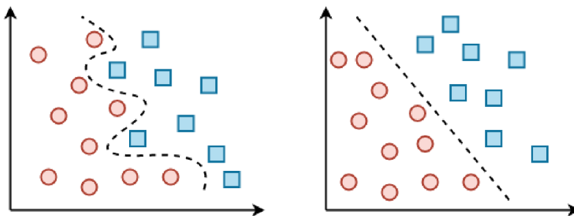
Obr. 4.4: Zobrazuje princíp transformácie dát do vyššej dimenzie, prevzané z [25]
