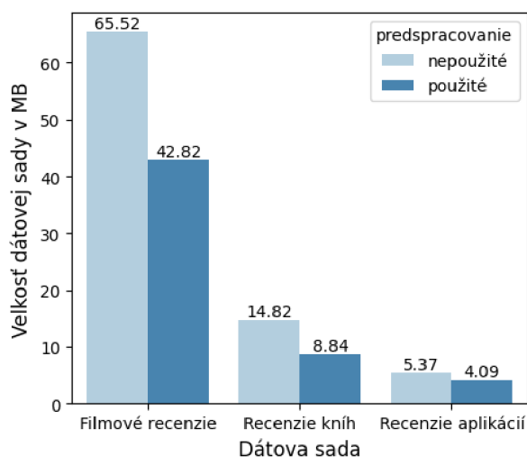
Obr. 6.3: Graf vplyvu predspracovania na veľkosť dátovej sady
