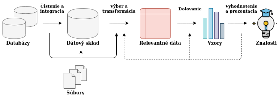
Obr. 2.1: Kroky procesu získavania znalostí, prevzaté z [26]
