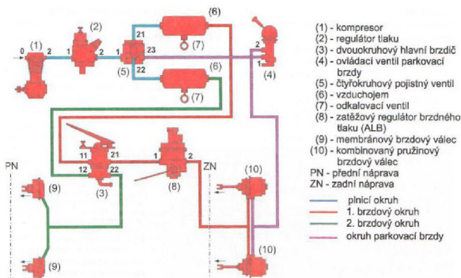
Obrázek 5.9: Dvouokruhová vzduchotlaká brzdná soustava [51]
