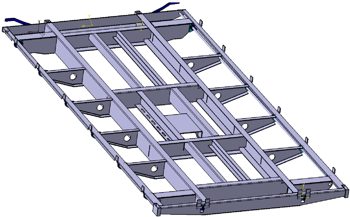
Obrázek 5.20: Rám korby
