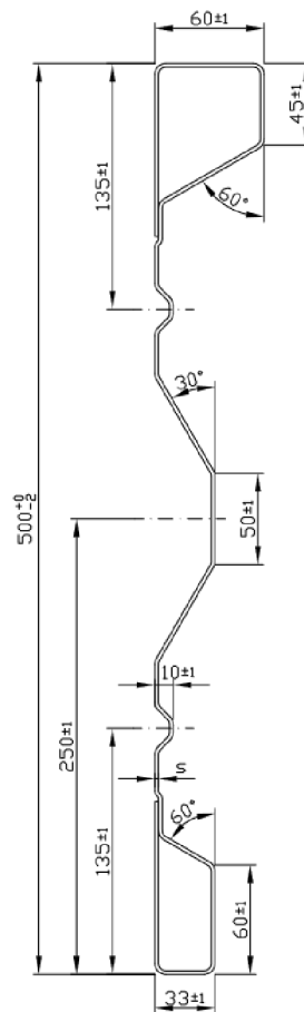
Obrázek 5.21: Profil bočnice [55]
