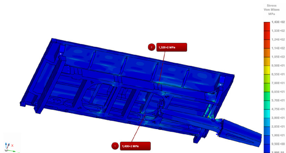
Obrázek 9.7: Napětí - HMH (top, bottom), konstrukce rámu - akcelerace návěsu, stupnice 0 – 143\text{ MPa}
