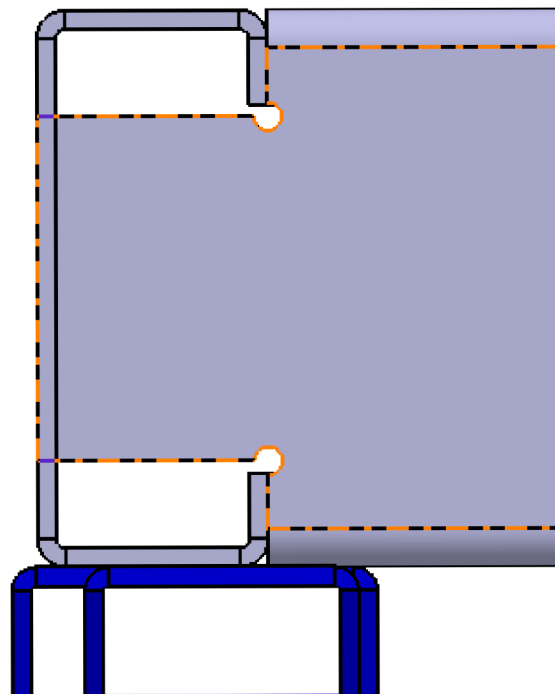
Obrázek 5.3: Způsob kolmé svařování profilů pro dynamicky namáhané svarky
