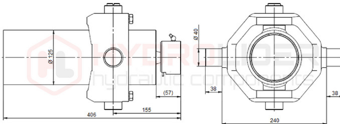
Obrázek 5.10: Hydraulický píst s klecí [52]
