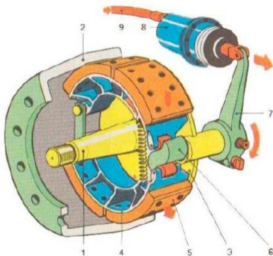
Obrázek 3.20: Bubnová brzda vzduchotlaká. 1-čep kola, 2-brzdňý buben, 3-štit brzdny, 4-brzdňá čelist, 5-brzdňé obložení, 6-brzdňý "S"klíč, 7-brzdňá páka, 8-pístový brzdňý váleček, 9-přívod tlakověho vzduchu [43]
