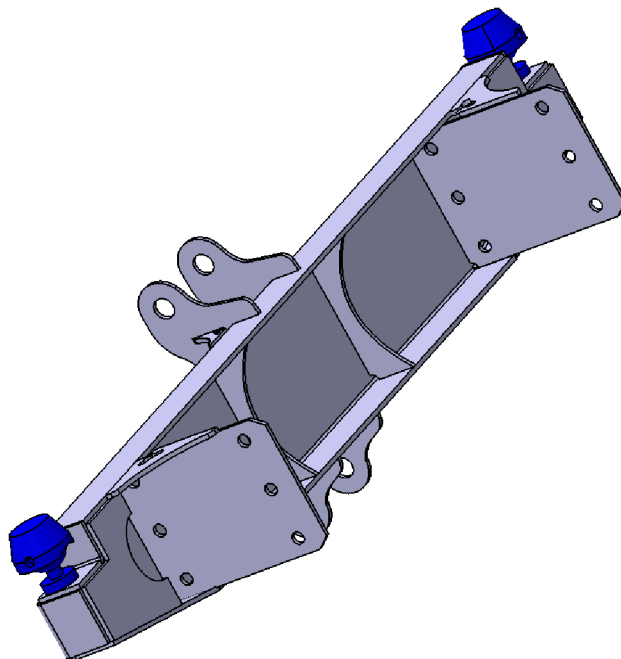
Obrázek 5.1: Přední část rámu návěsu
