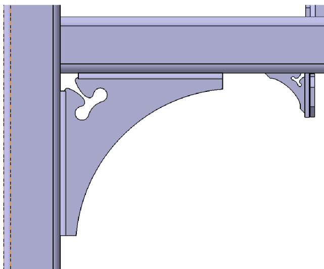
Obrázek 5.4: Konstrukční řešení pro rozložení napětí kolmého svaření profilů
